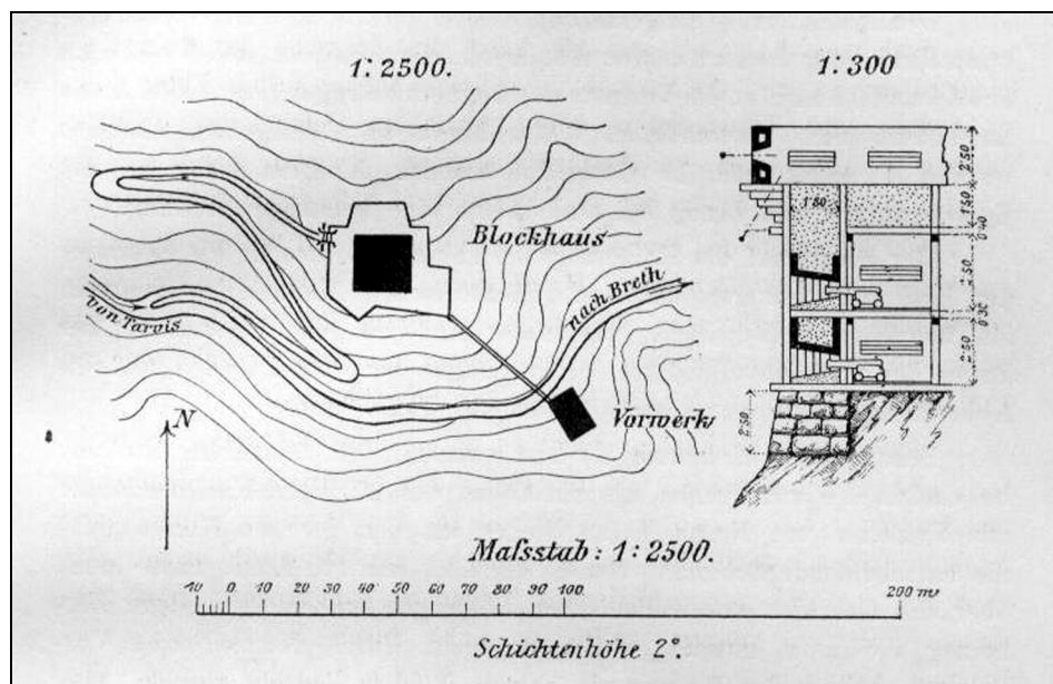
Sl. 5. Austrijska utvrda na Predilu (V. Klavara, 2003, 195).
