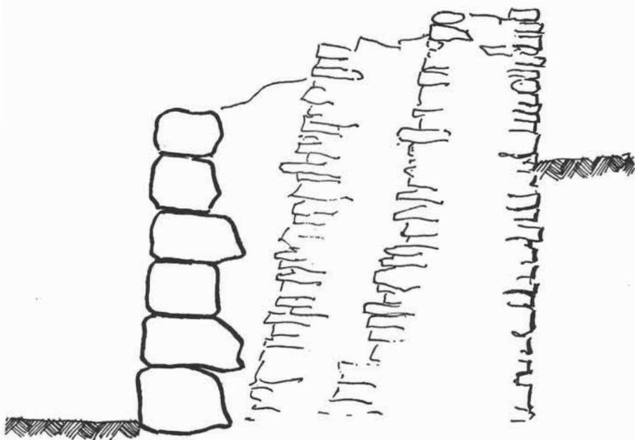
Sl. 3. Presjek bedema na zapadnoj strani: red bunja s vanjskog lica i dvostruki zaključeni zidovi u zidnoj postavi
