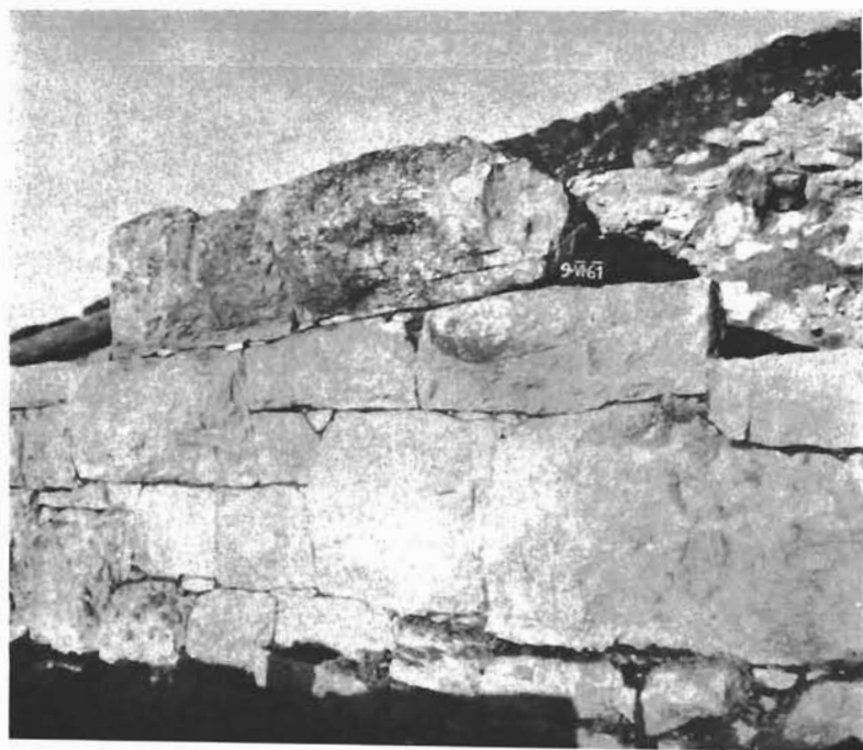
Sl. 1. Struktura bunja u bedemu na zapadnoj strani u fazi otkrivanja
