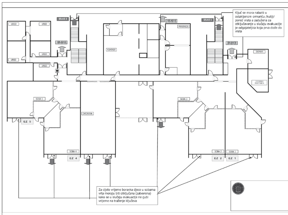
Slika 1. Evakuacijska shema (prizemlje)
