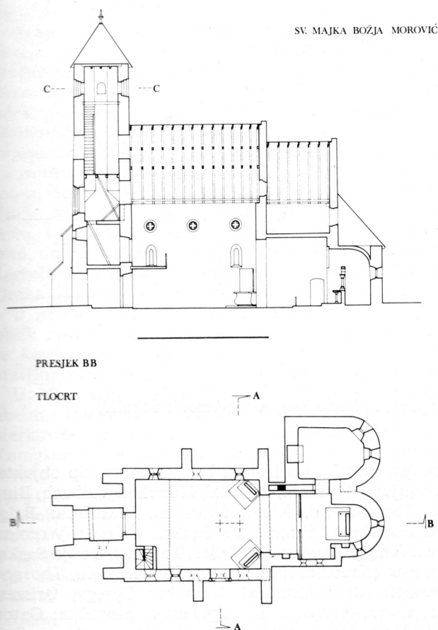
2 Tlocrt i presjeci crkve u Moroviću (arh. snimak Sena Gvozdanović-Sekulić)
