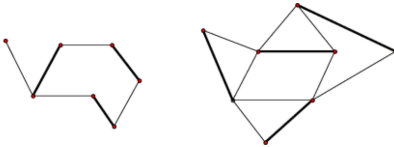
Slika 1: Primjer maksimalnog i savršenog sparivanja
