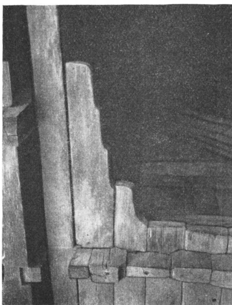
Kuća Posilović u Martinskoj Vesi desnoj — detalj konstrukcije za podupiranje gornjeg poda.
