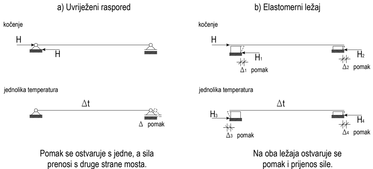
Slika 4 – Prijenos sila i pomaka
