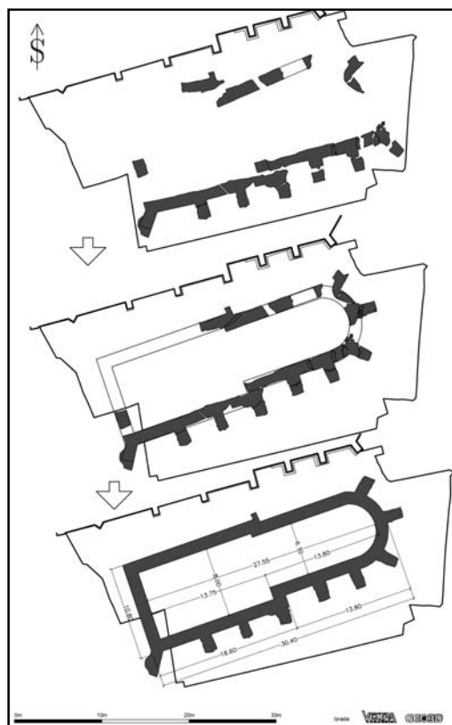
Remete, samostan Blažene Djevice Marije. Tlocrt zatečenog stanja, tlocrt stanja nakon spajanja i kotirani tlocrt idealne rekonstrukcije druge građevinske faze samostanske crkve. Izrada: Vektra-Geo3D.
