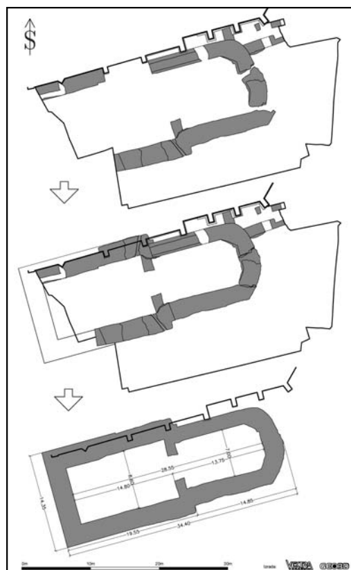
Remete, samostan Blažene Djevice Marije. Tlocrt zatečenog stanja, tlocrt stanja nakon spajanja i kotirani tlocrt idealne rekonstrukcije prve građevinske faze samostanske crkve. Izrada: Vektra-Geo3D.
