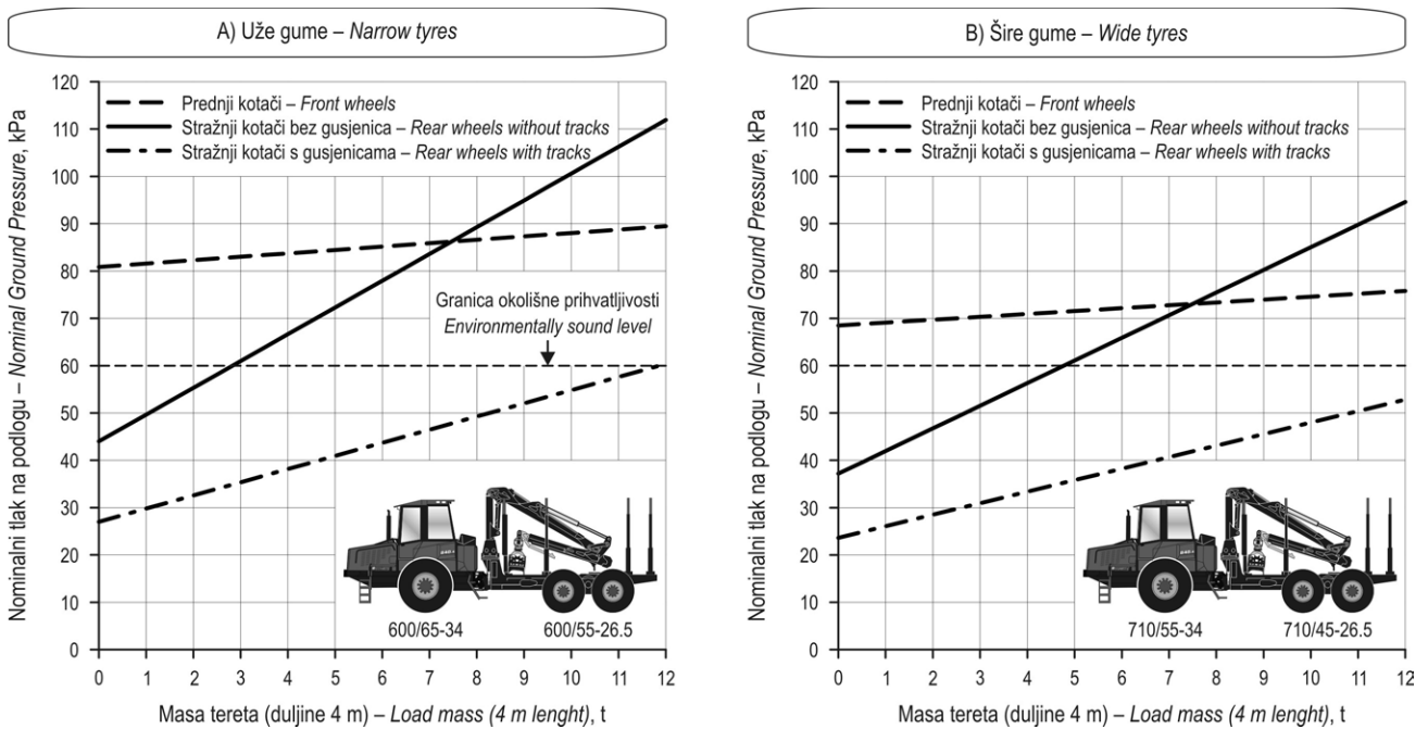
Slika 7. Ovisnost nominalnoga tlaka prednjih i stražnjih kotača (gusjenice) ovisno o masi utovarenoga drva
