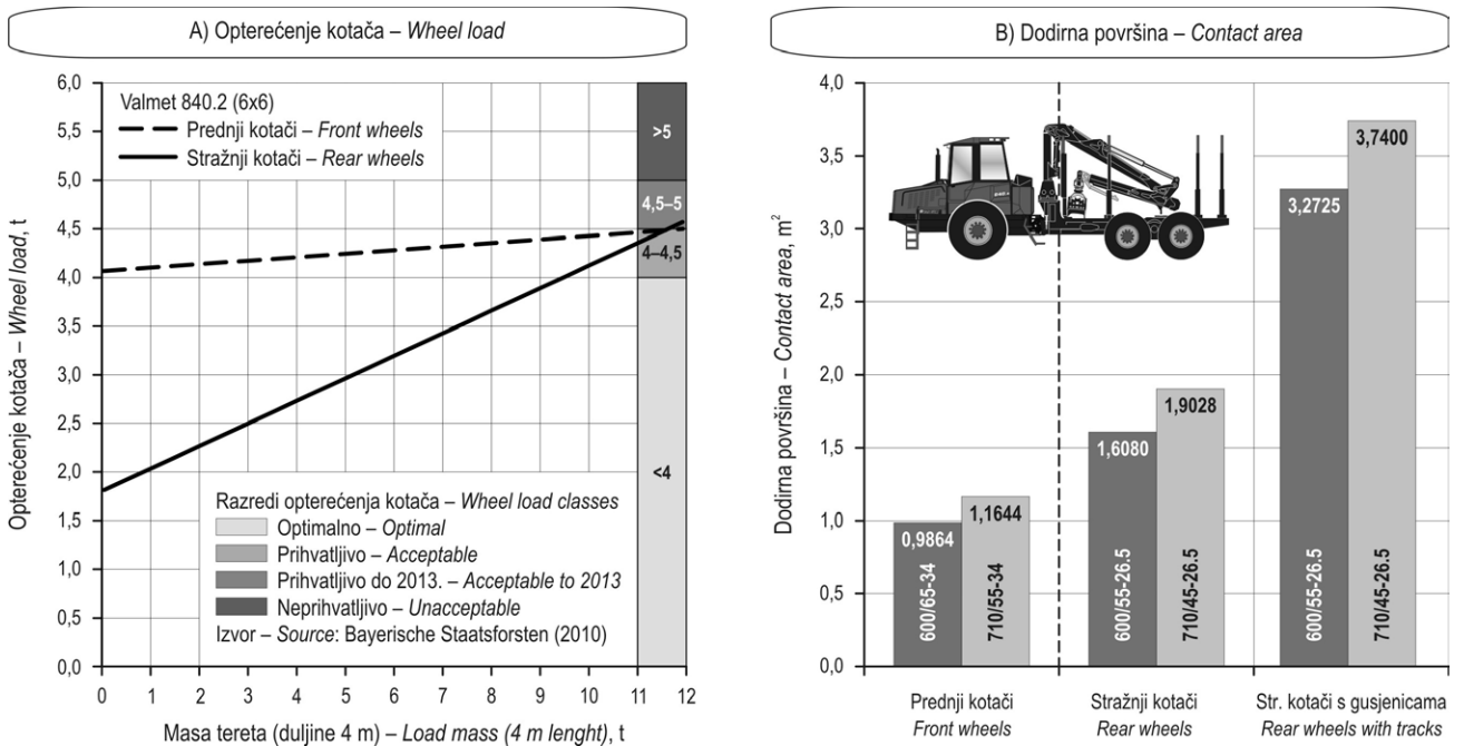
Slika 6. Opterećenje kotača i dodirna površina forvardera Valmet 840.2 (6 × 6)
