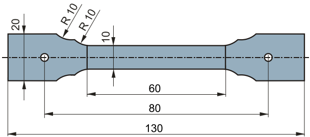
Figure 2. Tensile test bar Slika 2. Ispitivana epruveta
