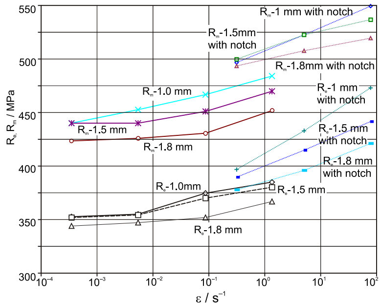
Figure 7. Influence of the strain rate \epsilon on the yield point R_e and the tensile strength R_m of the tested sheets Slika 7. Utjecaj brzine deformacije \epsilon na granicu razvlačenja R_e i vlačnu čvrstoću R_m ispitivanih traka
