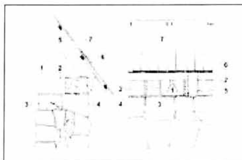
Sl. 8. Detalj krovnog veza: 1-vezna greda 22/30, 2-"coljak" 22/30, 3-"podzidnica" 22/30, 4-jasenov klin, 5-rog 14/16, 6-krovnna letva, 7-šimla
