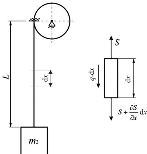
Figure 7 Oscillation of a rope with constant length Slika 7. Oscilacije užeta sa stalnom dužinom
