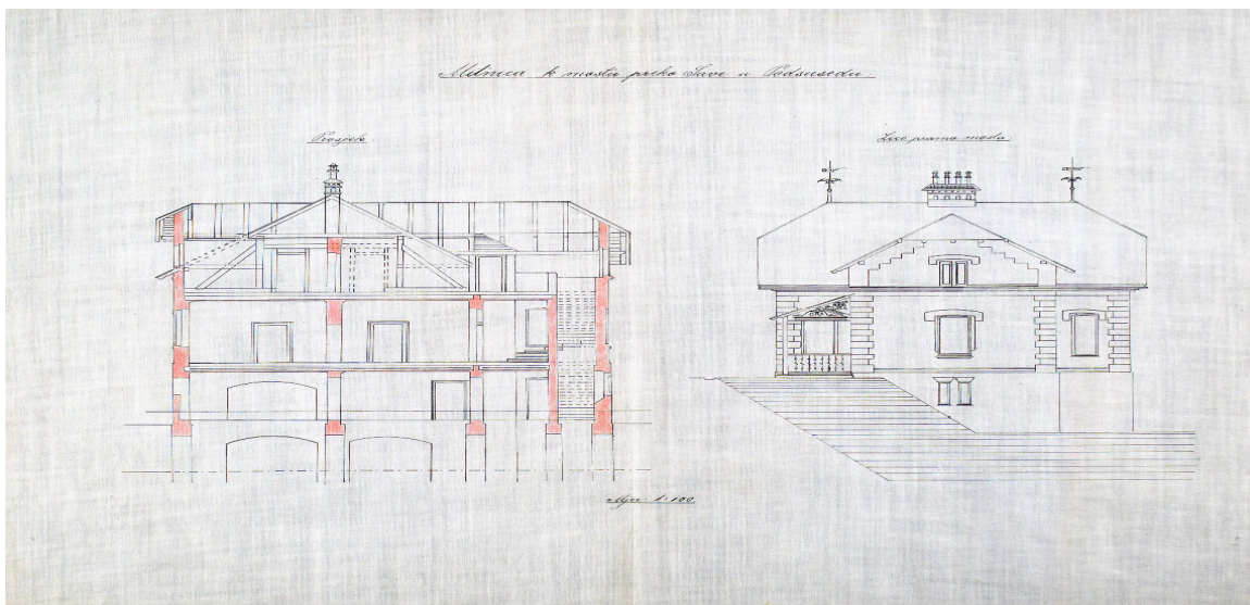
Mitnica na mostu preko Save kod Podsuseda - nacrt, UOZV, sv. X 317/1899 (42516/1899), fragment 3
