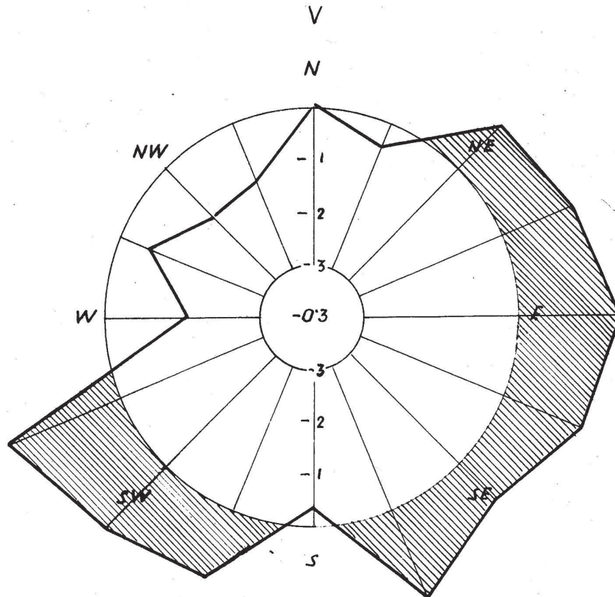
SL.2.2.3(vi). SREDNJA TERMIČKA RUŽA VJETRA U JESEN ; LUČKO 1949/55.
