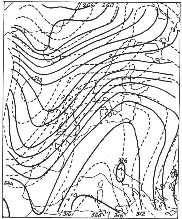
SL.3.3.2.1.(vi). RT 700 500 20.XII.1951. 03h RT 1000
