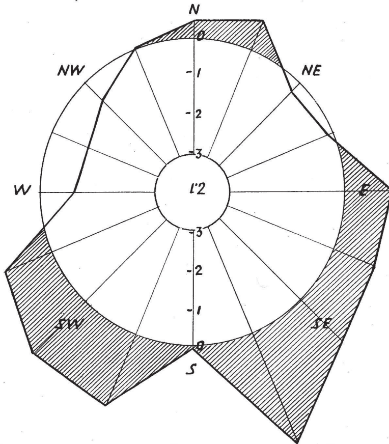
SL.2.23.(ii). SREDNJA GODIŠNJA TERMIČKA RUŽA VJETROVA LUČKO 1949-1955
