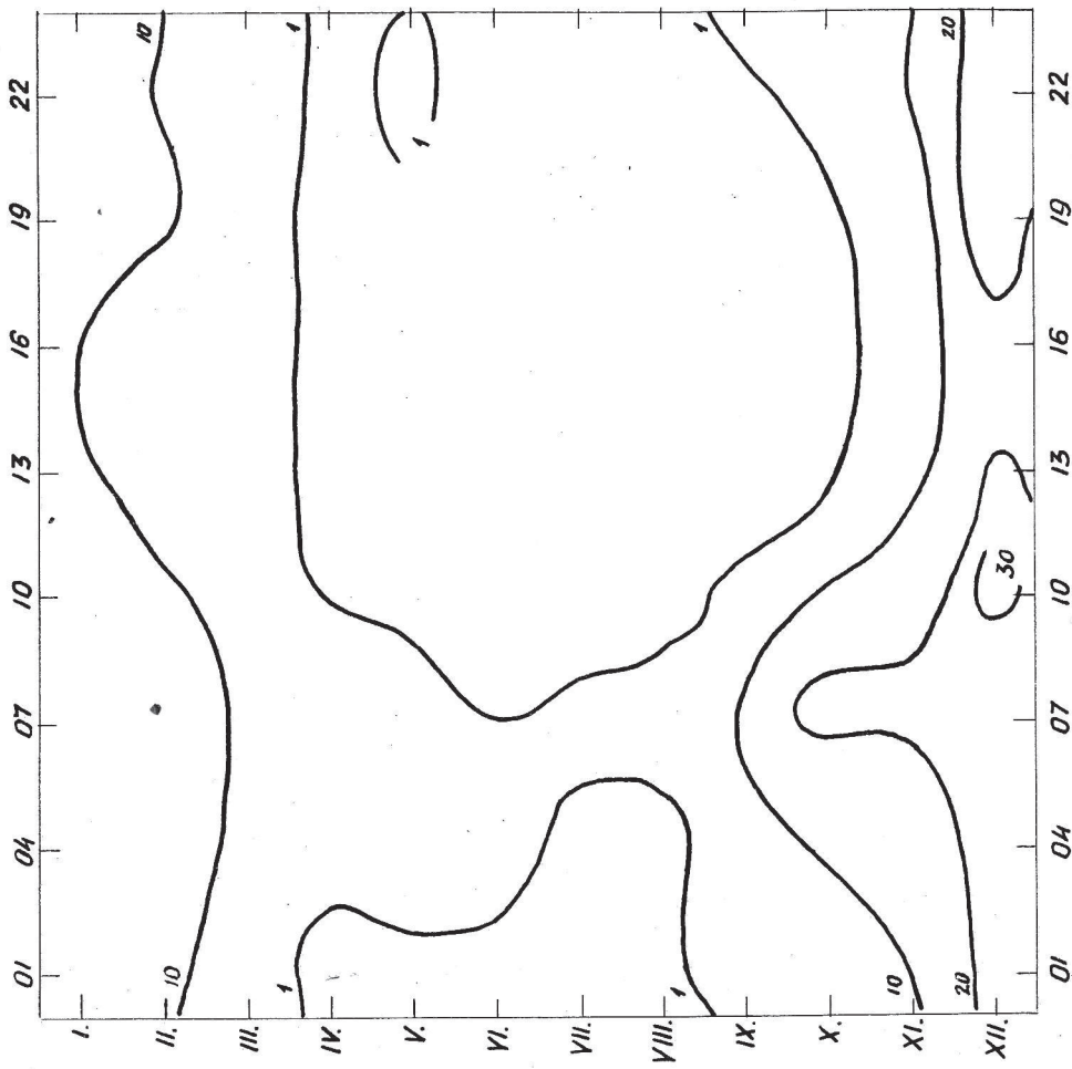
Sl. 3.2.7.(ž). Izoplete prilika lošeg vremena na Lučkom 1949 - 1955.
