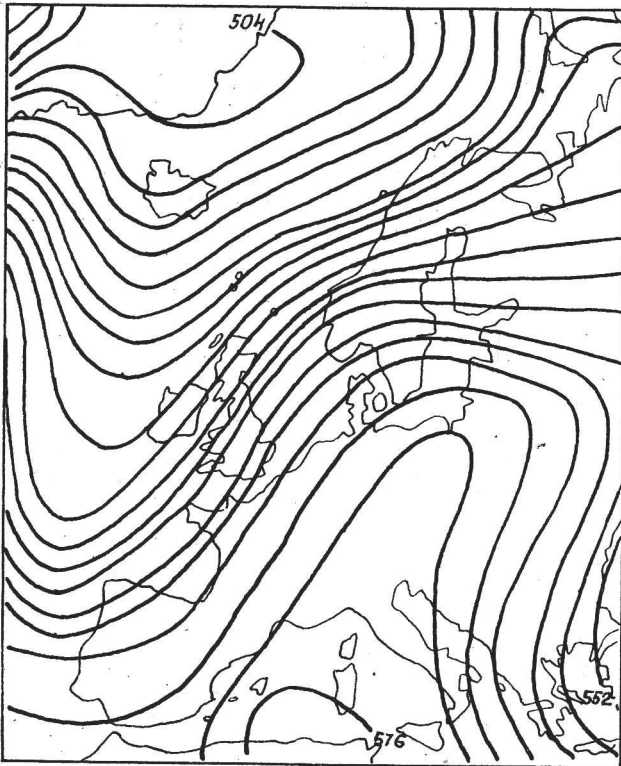
SL.3.3.2.1.(V). RT 500 20.XII.1951. 03h
