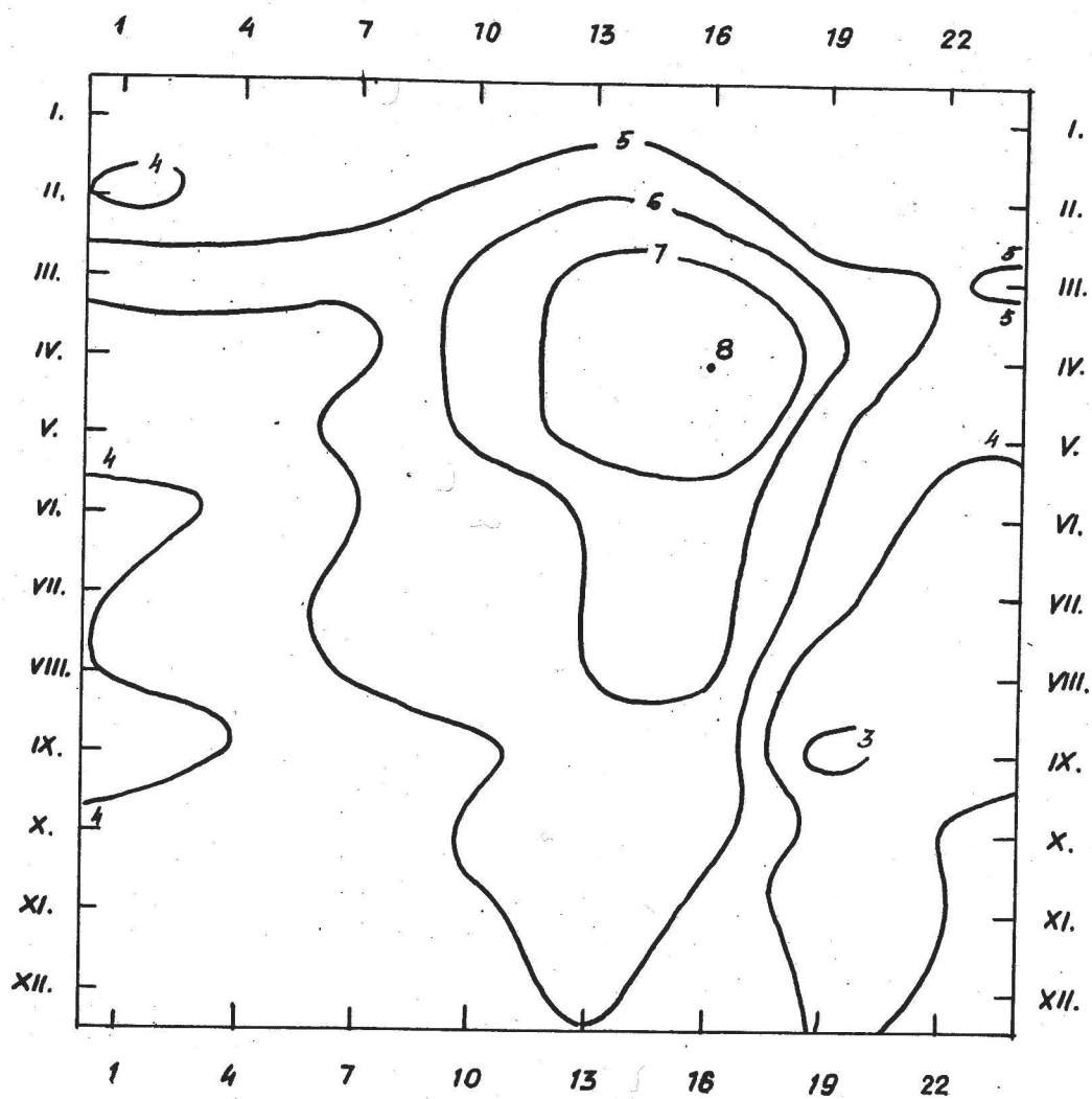
SL.5.2.(i). IZOPLETE SREDNJE BRZINE VJETRA U ČV. LUČKO 1949-1955.
