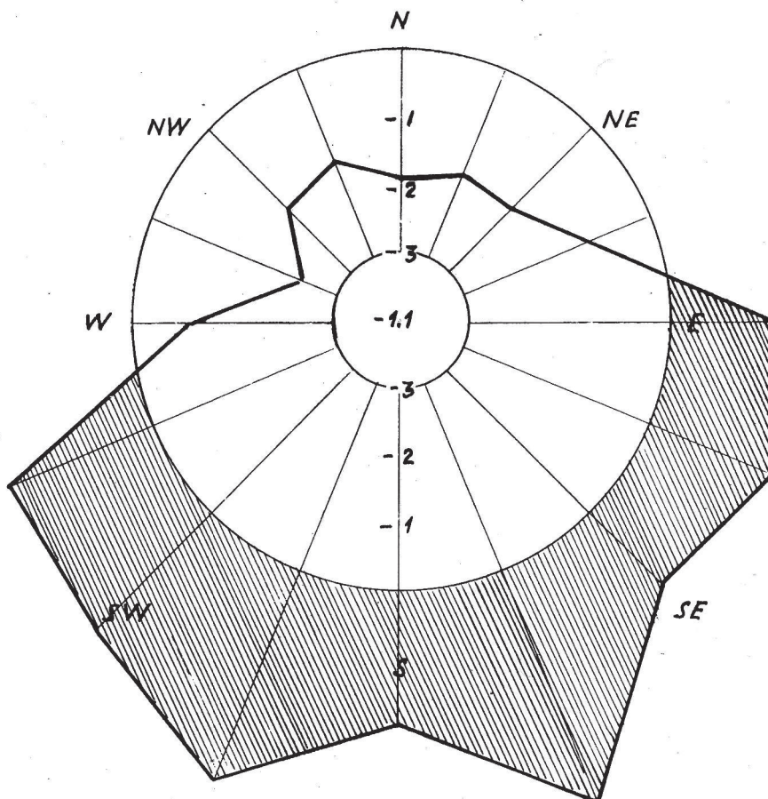
SL. 22.3.(iv). SREDNJA TERMIČKA RUŽA VJETRA U PROLJEĆE LUČKO 1949.-1955.
