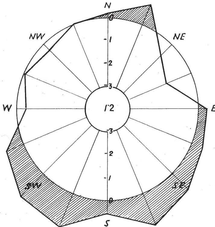
SL.2.23.(iii). SREDNJA TERMIČKA RUŽA VJETROVA ZIMI LUČKO 1949-1955.
