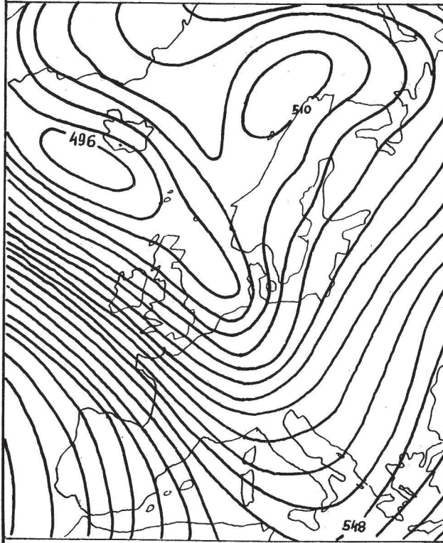
SL.3.3.2.2(xi). RT 500 1.11.1952. 03h
