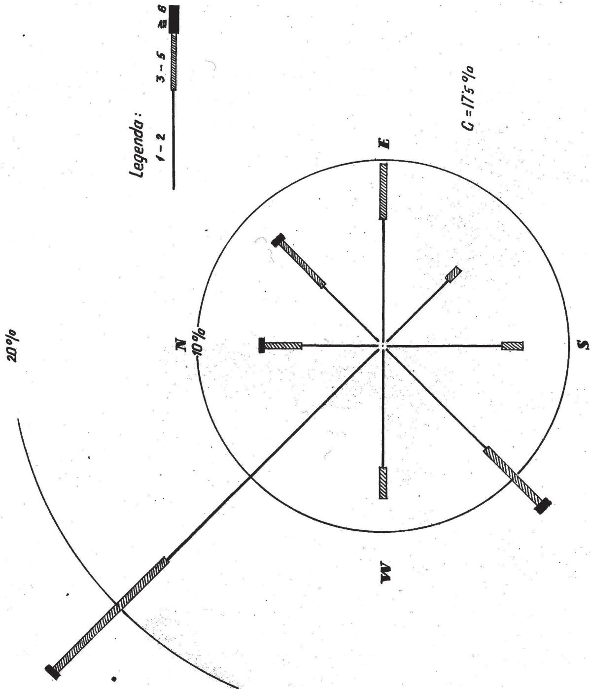
SL. 5.3. (i). SPREDNJA GODIŠNJA RAZDIJELA SMJEROVA VJETRA NA LUČKOM (1945-1955.)
