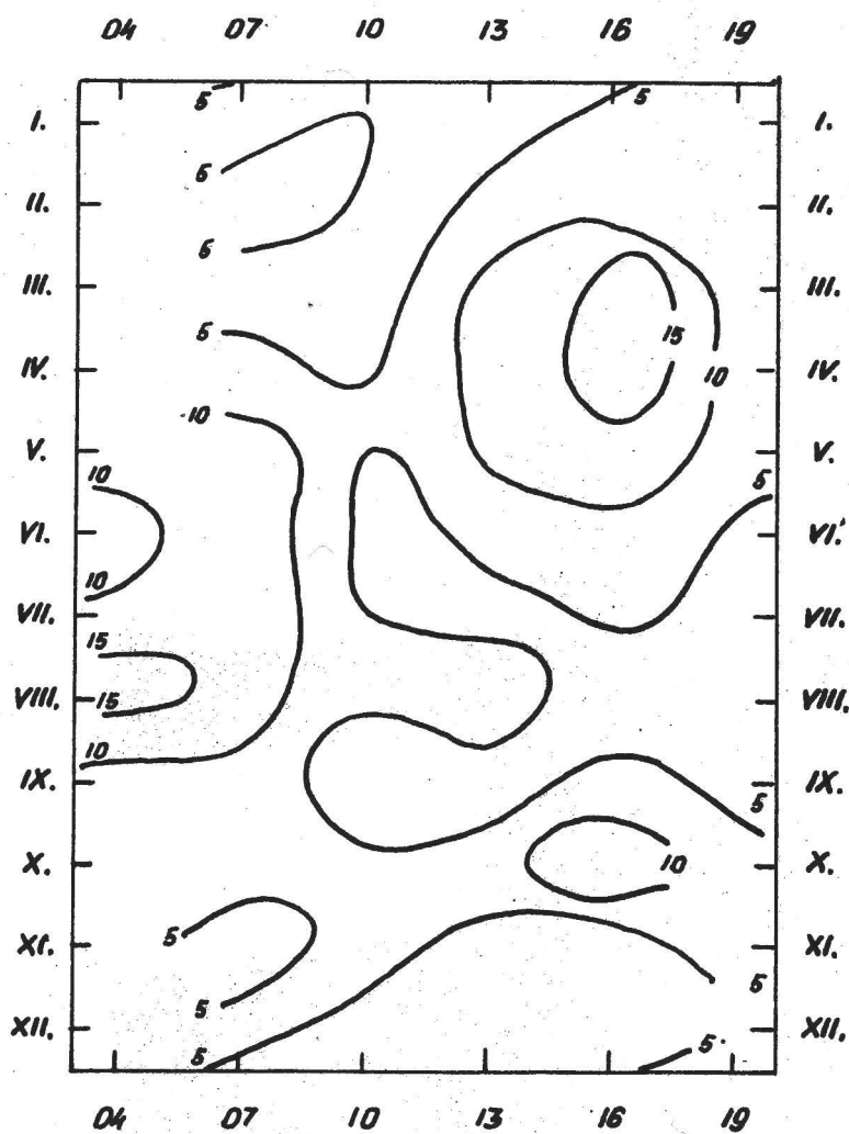
SL. 5.4.2 (1). IZOLETE RAZLIKE ČESTINA NAJPOVOLJNIJEG I NAJNEPOVOLJNIJEG PRAVCA UZ KRITIČNU BRZINU 10 mi/h. LUČKO 1949-1955
