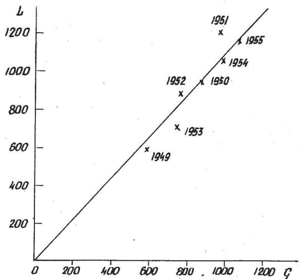
SL. 2.4.1. (i). VEZA IZMEĐU GODIŠNJE KOLIČINE OBORINE NA LUČKOM I OPSERVATORIJU ZAGREB-GRİČ 1949 - 1955.
