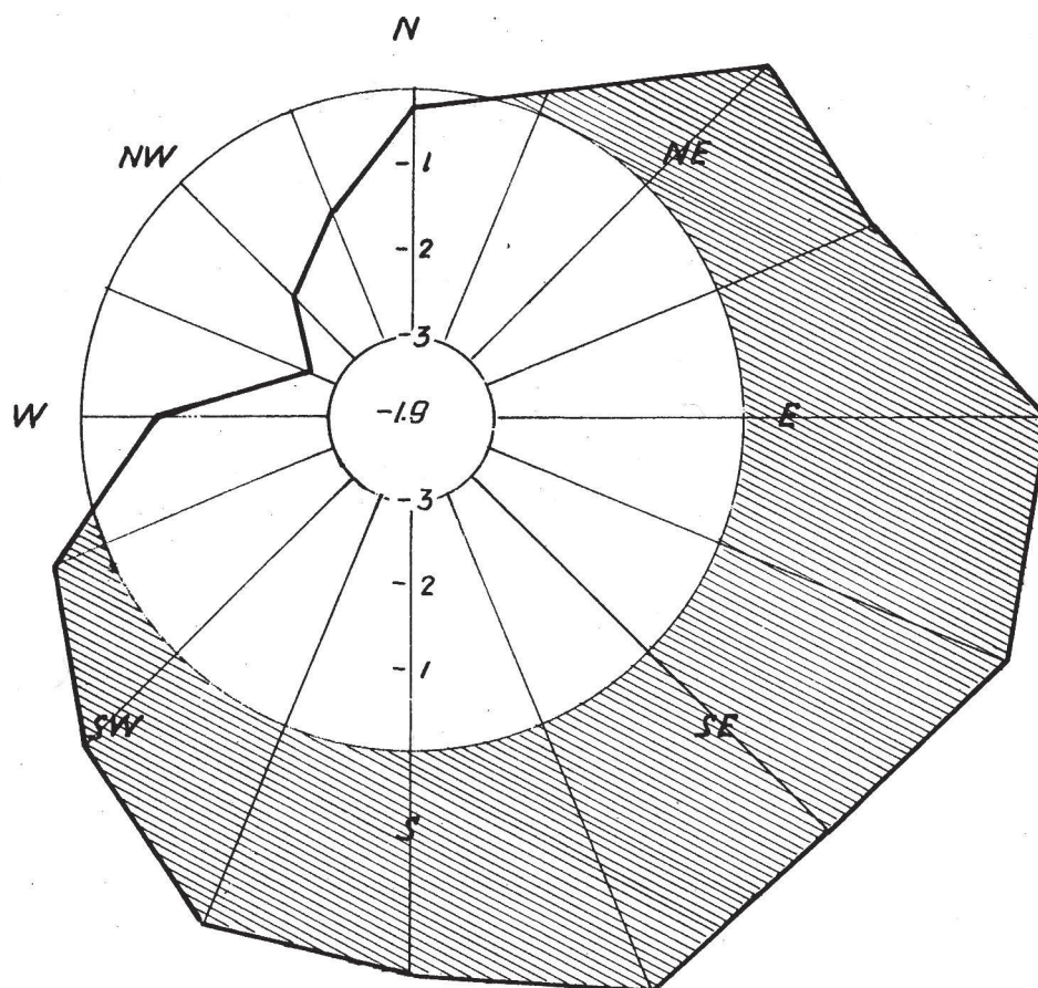
SL. 22.3(v). SREDNJA TERMIČKA RUŽA VJETRA LJETI LUČKO 1949.-1955.
