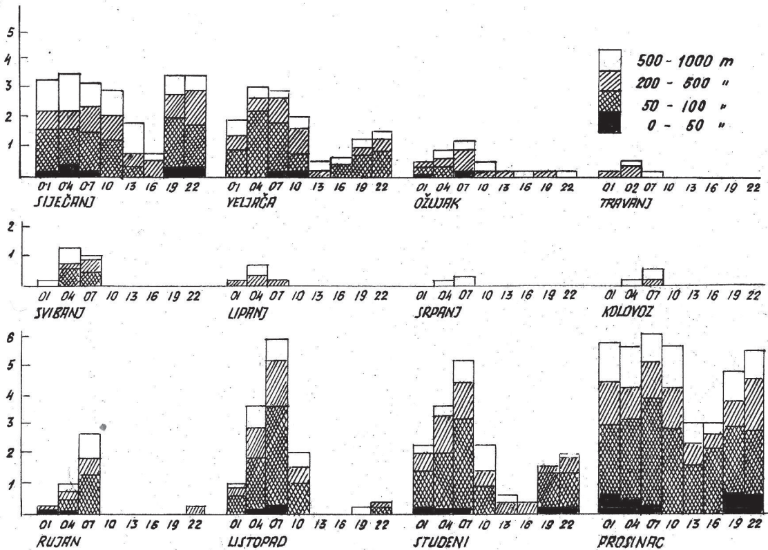
SL. 3.2.2.(vi). RAZDIJELA MAĞLE PO JAČINI ZA MJESEGE I TERMINE LUČKO 1949/55.
