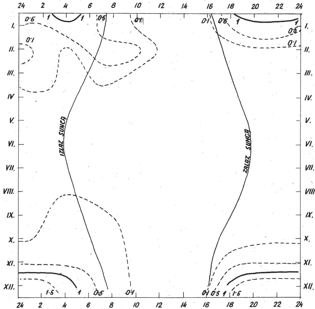
SL. 3.2.2(v). IZOLETE VJEROJATNOSTI (%) MAĞLE (V < 50 m) NA LUČKOM 1949./55.
