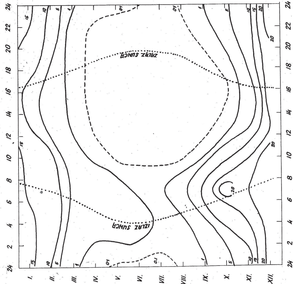
SL. 3.2.2. ( ž ). IZOPLETE VJEROJATNOSTI (%) MAĞLE ( V < 2 km ) NA LUČKOM 1949 - 1955.
