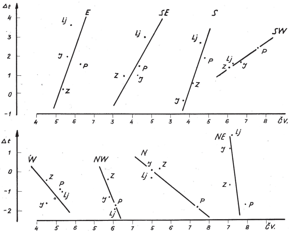
SL.2.2.3.(vii). ZAVISNOST TEMPERATURE O BRZINI I SMJERU VJETRA LUČKO 1949-1955.
