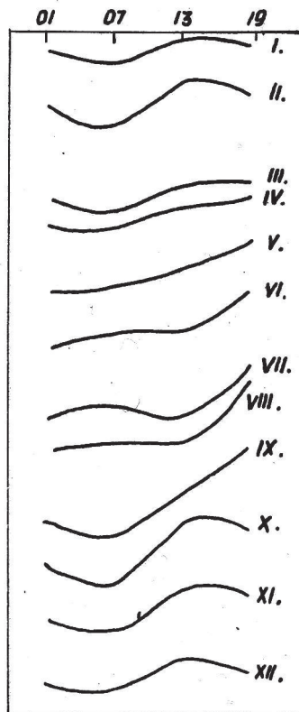
SL. 2.3.2. (ii). SREDNJI DNEVNI HOD OMJERA MIJEŠANJA LUČKO 1949-1955.
