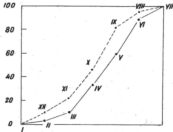
SL. 2.3.2 (i). SREDNJI GODIŠNJI HOD RELATIVNOG OMJERA MIJEŠANJA LUČKO 1949-1955.
