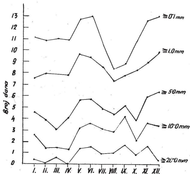
SL. 2.4.2. (i). SREDNJI GODIŠNJI HOD BROJA DANA S OBORINOM NA LUČKOM 1949 - 1955.
