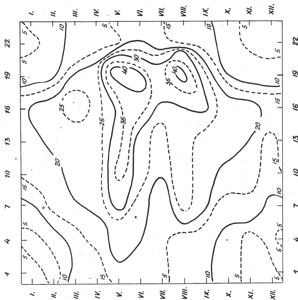
SL.4.2.(ii). IZOPLETE VJEROJATNOSTI POJAVE RODA OBLAKA Ci NA LUČKOM 1949-55.
