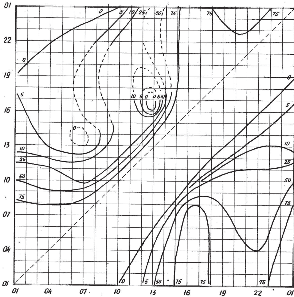
SL. 3.2.2. (xiii). GRAFIKON ZA ODREĐIVANJE VJEROJATNOSTI TRAJANJA MAGLE, LUČKO 1949/55. ( V < 2\text{Km} ) JESEN
