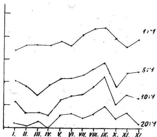
SL. 2.4.2. (ii). SREDNJI RELATIVNI GODIŠNJI HOD BROJA DANA S OBORINOM NA LUČKOM 1949 - 1955.
