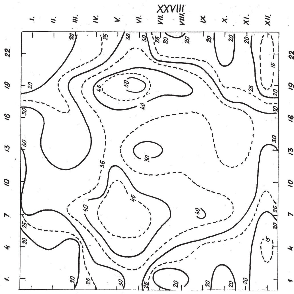
SL.4.2.(v).IZOPILETE VJEROJATNOSTI POJAVE RODA OBLAKA Ag LUČKO 1949-55.
