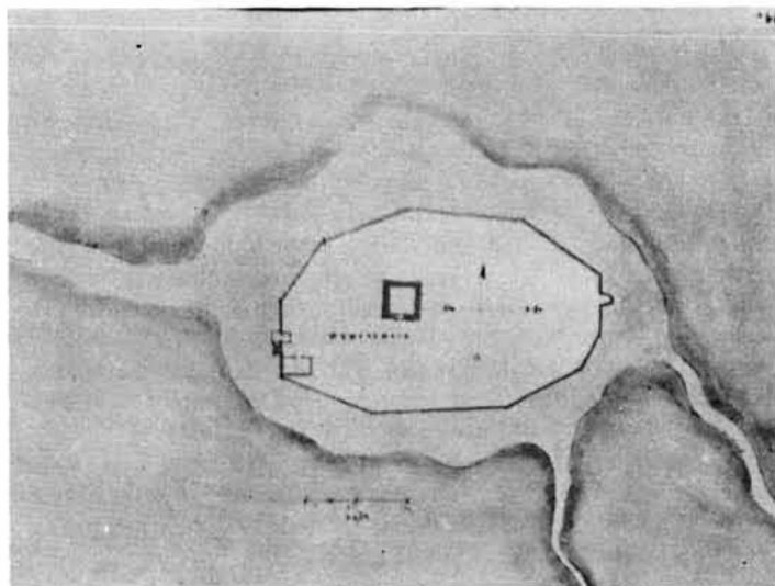
Sl. 27. – Otočac, utvrde grada pri kraju XVI. st. ÖNB, Wien, Cod.8609
