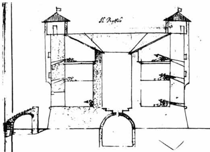
Sl. 26. – Senj, kula Nehaj, presjek tvrđave, AS., Reluzioni di anno 1639, G. Pieroni
