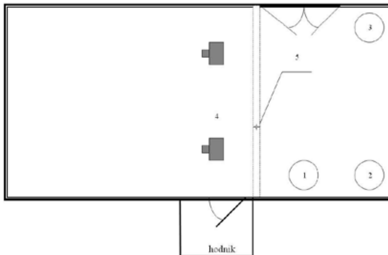
1, 2 i 3 – filter (spremnik); 4 – stup; 5 – ojačanje s metalnom vodilicom i pričvrsnim vijcima
