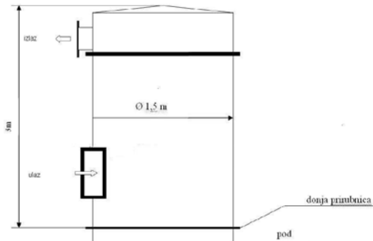
Slika 2. Filter (spremnik); (strelicama su na priрубnicama označeni smjerovi strujanja zraka - ulaz i izlaz)
