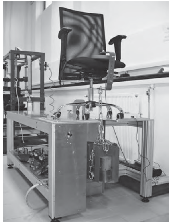
Stol za ispitivanje stabilnosti uredskih, školskih i drugih vrsta stolica
