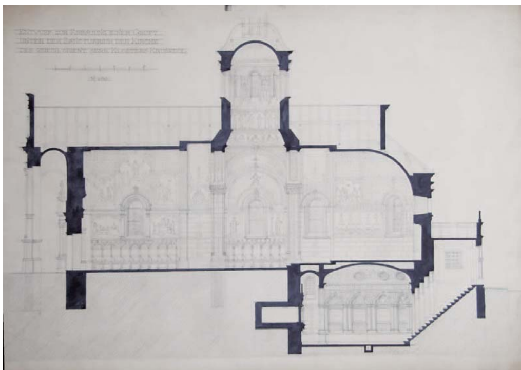
4. Herman Bollé, Prva varijanta projekta za izgradnju kripe u crkvi manastira Krušedola, uzdužni presjek, 1901., NAZ, ZGN, sign. II-29.
