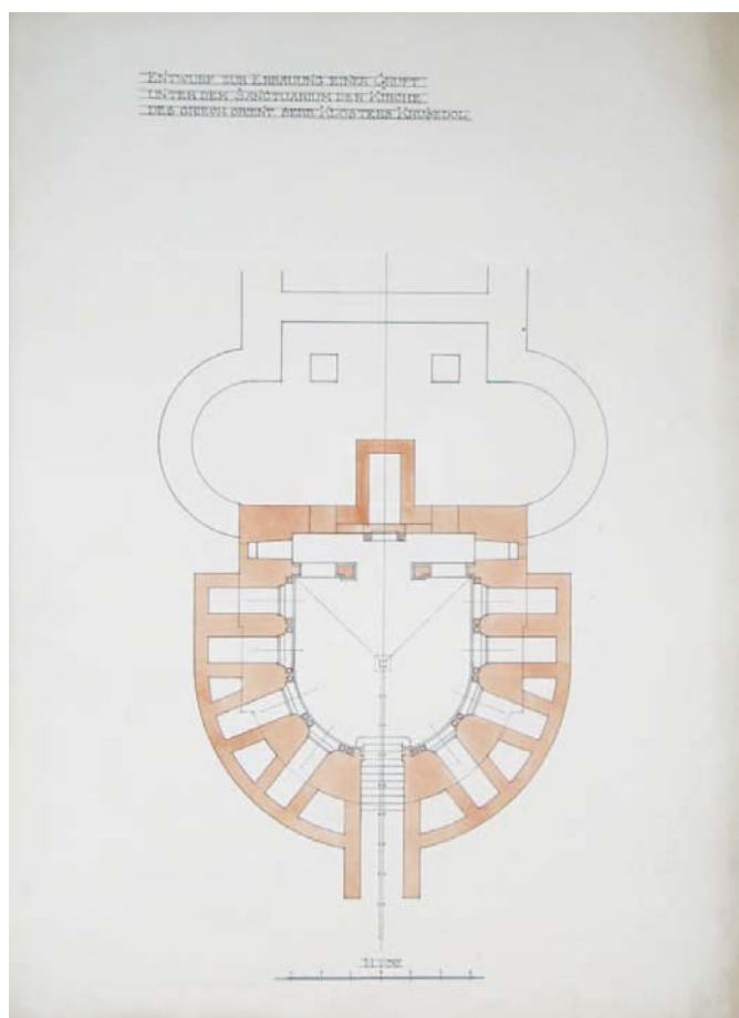
6. Herman Bollé, Prva varijanta projekta za izgradnju kripe u crkvi manastira Krušedola, tlocrt, 1901., NAZ, ZGN, sign. II-29.
