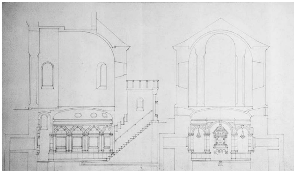
5. Herman Bollé, Prva varijanta projekta za izgradnju kripe u crkvi manastira Krušedola, poprečni i uzdužni presjek, 1901., NAZ, ZGN, sign. II-29.
