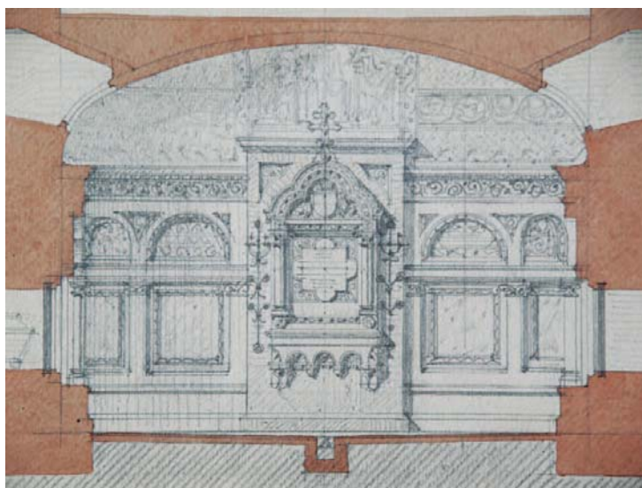
8. Herman Bollé, Druga varijanta projekta za izgradnju kripe u crkvi manastira Krušedola, poprečni presjek, detalj s prikazom zida na kojemu se trebao nalaziti spomenik kralja Milana, 1902., NAZ, ZGN, sign. II-29.
