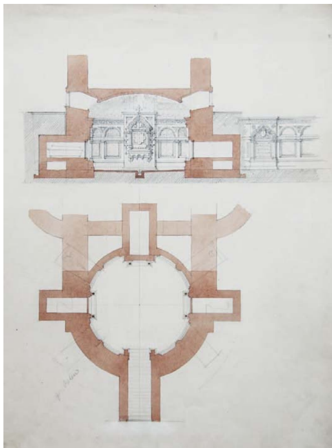
7. Herman Bollé, Druga varijanta projekta za izgradnju kripe u crkvi manastira Krušedola, tlocrt i poprečni presjek, 1902., NAZ, ZGN, sign. II-29.
