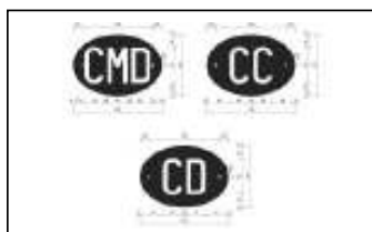
Slika 4: Dopunske pločice
