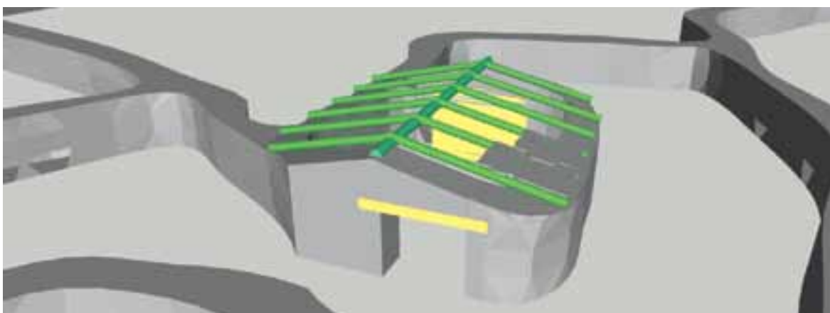
Sl.6. Konstruktivni elementi nastambe na Starom Raklju
