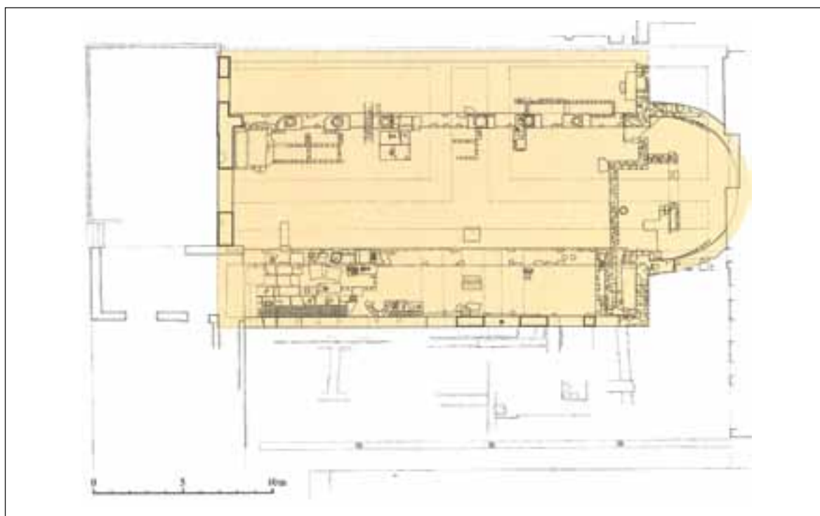
Sl. 6. Bazilika sv. Tome, tlocrt arhitektonskih ostataka (preuzeto: VEŽIĆ, 2005.)
