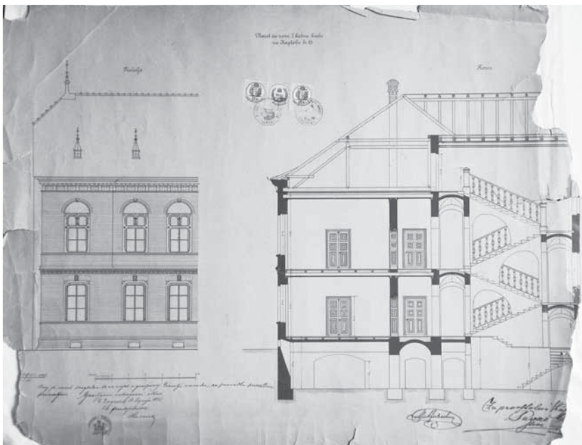
H. Bollé, Projekt za glavno pročelje i presjek kurije Kaptol 21, 1885. (NAZ, Zbirka građevnih nacрта, sign. III-15)
