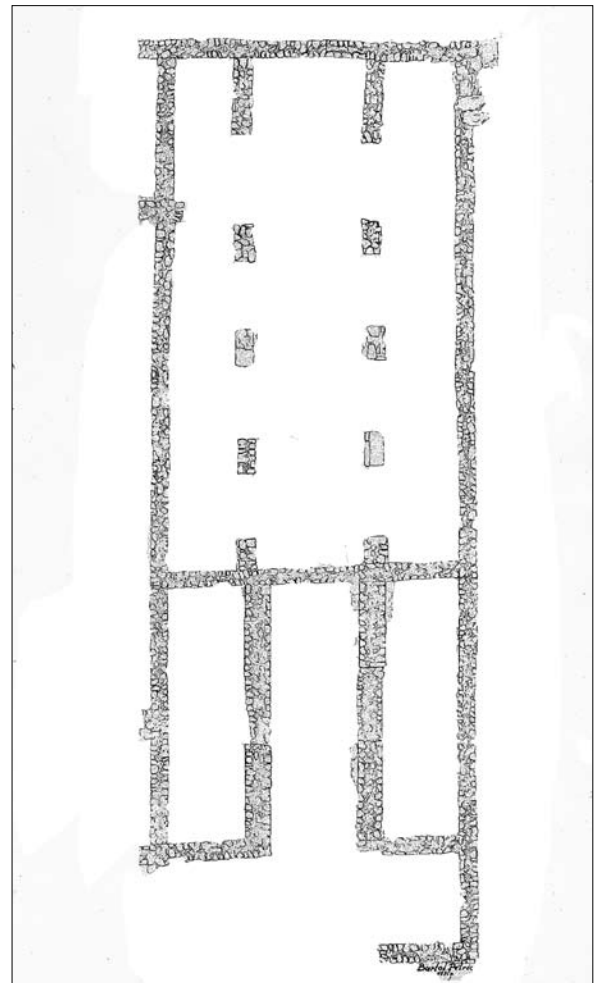
Tlocrt br. 4, Crkva u Biskupiji kod Knina
