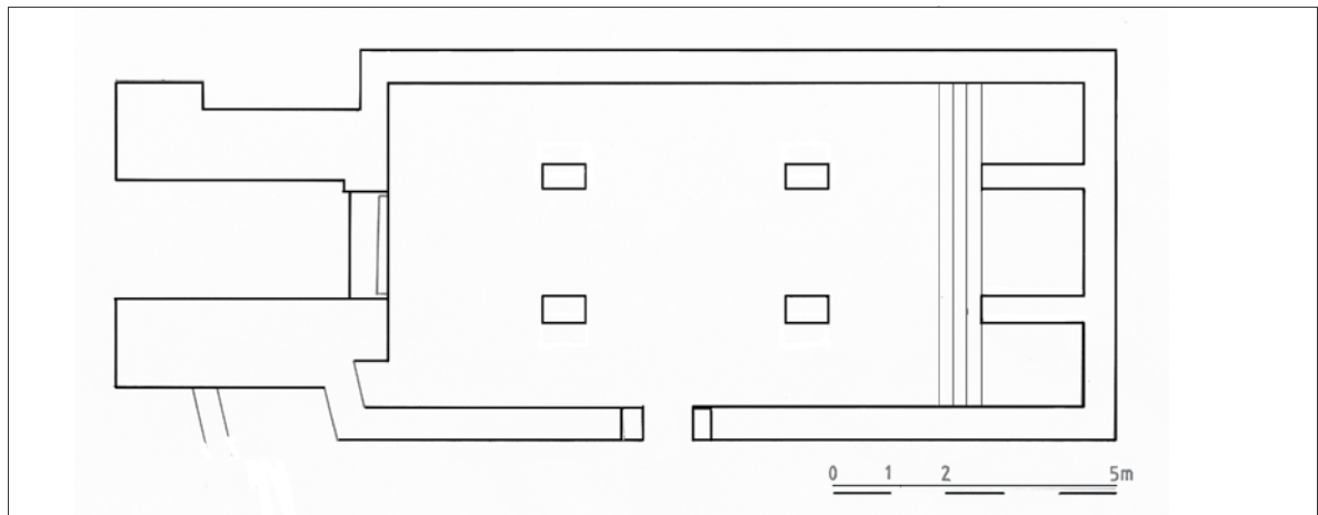
Tlocrt br. 3, rekonstrukcija A. Jurčević
