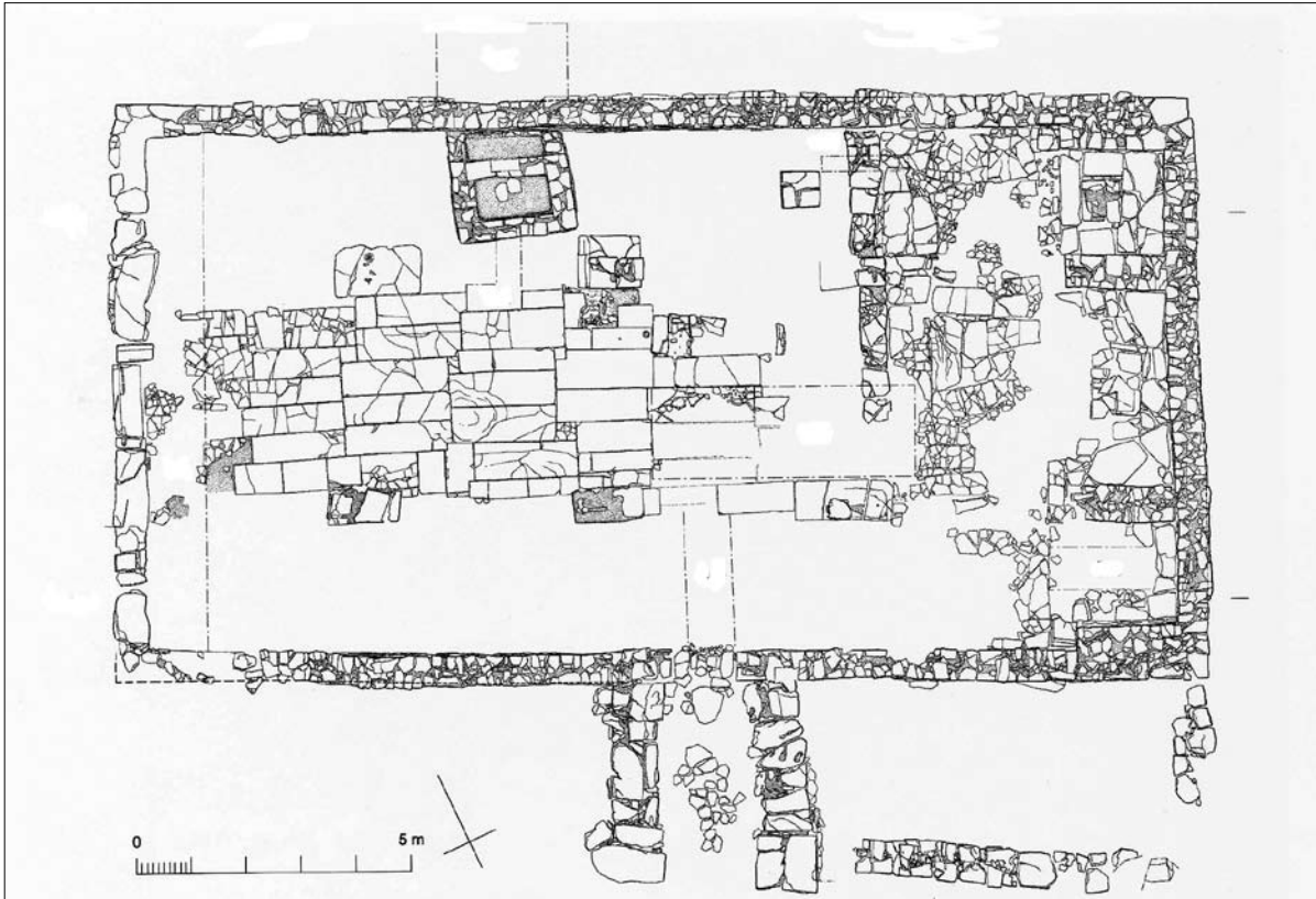
Tlocr br. 5, trobrodna bazilika u Guranu
