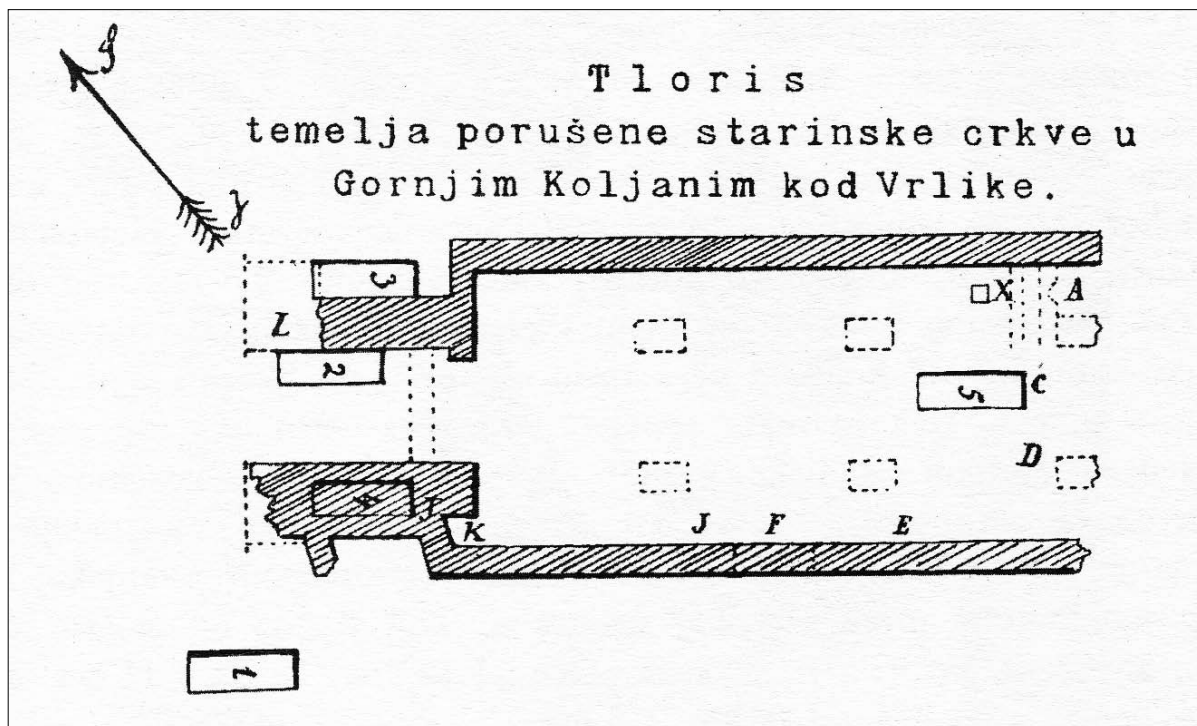
Tlocrt br. 1, donosi ga F. Radić 1900. g.
