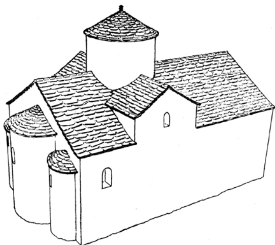
Sl.7 Pretpostavljeni izvorni izgled crkve (J. Marasović)
