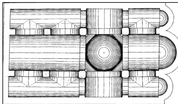
Sl. 8 Pretpostavljeni tlocrt svodova crkve (J. Marasović)
