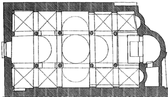
Sl.13 Tlocrt crkva S. Giovanni a mare u Gaeti
