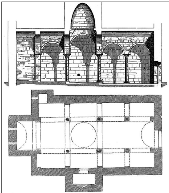
Sl. 3 Zimmermannovi snimci crkve, koje je objavio Eitelberger 1861.
