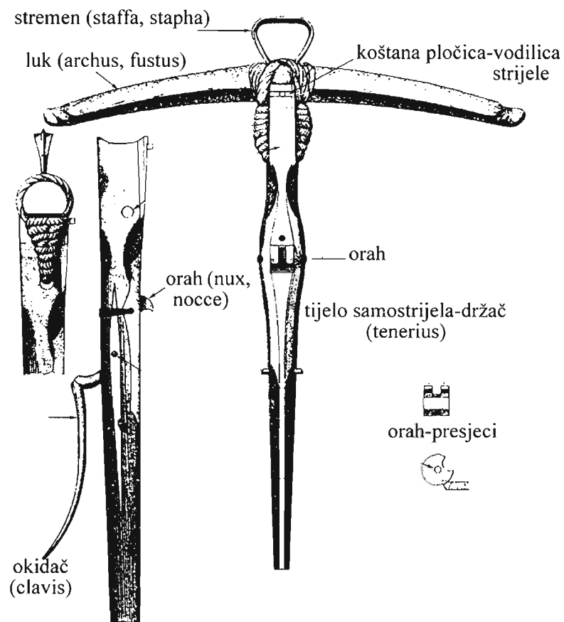
Sl. 1. Osnovni dijelovi samostrijela
