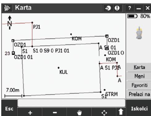
Slika 3.5. Prikaz izmjere željezne ograde
