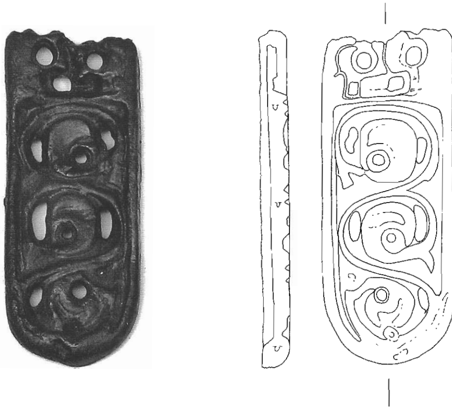
Sl. 1. Pojasni jezičac s motivom stilizirane krugolike lozice (foto: T. Sesar, crtež: Z. Podrug)
