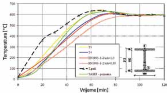
Slika 15. Usporedba temperatura u elementu za nelinearnu krivulju zagrijavanja (600°C, test ekscentrični tlak)
