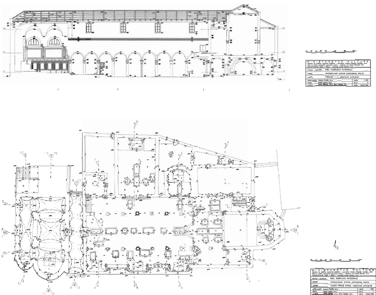
sl. 1 - Tlocrt i presjek katedrale sv. Marije i dvokatne crkve sv. Kvirina (snimili: S. Purišić d.i.a. i M. Lubina d.i.a.)
