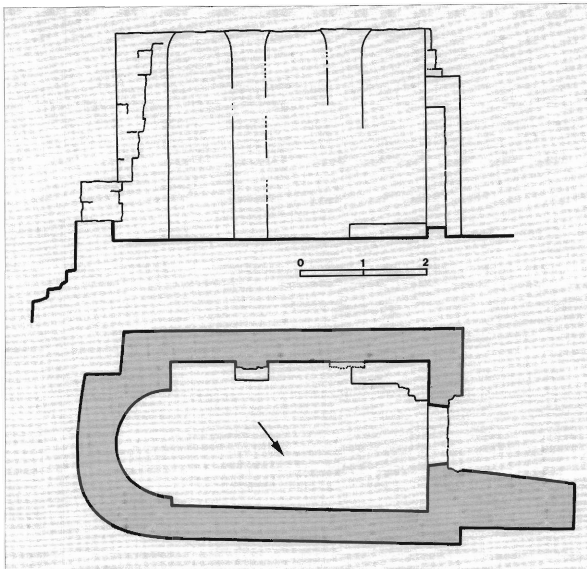
Crtež 1. Uzdužni presjek i tlocrt Sv. Martina, konzervatorski zahvat Instituta za povijest umjetnosti u Zagrebu (snimak I. Tenšek).
