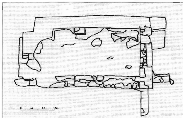
Crtež 1. Uzdužni presjek i tlocrt Sv. Martina, konzervatorski zahvat Instituta za povijest umjetnosti u Zagrebu (snimak I. Tenšek).
