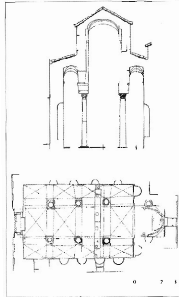
Presjek i tlocrt crkve Sv. Barbare u Trogiru (prema R. Bužančiću).
