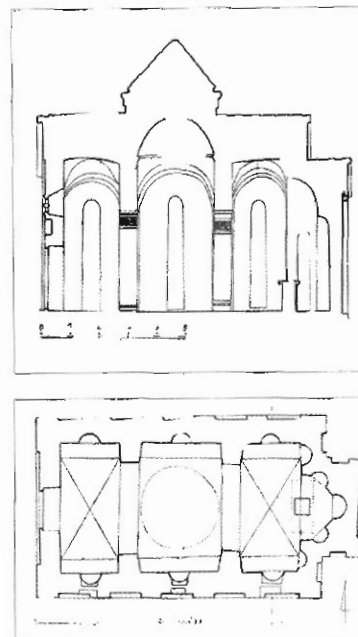
Presjek i tlocrt crkve Sv. Petra na Prikome u Omišu (D. Domanić).
