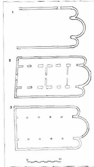
Tlocrti crkava iz doba kralja Petra Krešimira IV Sv. Petar u Osoru, Sv. Marija u Ninu Sv. Marija u Zadru, (I. Tenšek)
