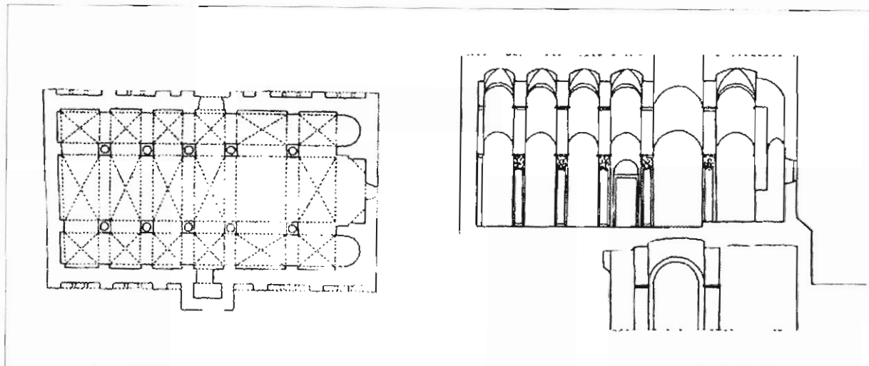
Tlocrt i presjek crkve St. Nedeljice u Zadru (prema P. Vežiću).
