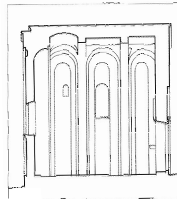
Poprečni i uzdužni presjek crkve Sv. Mihovila u Stonu (I. Tenšek).
