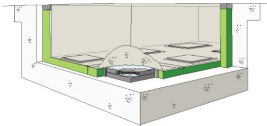
Slika 10. Izolacija temelja [6]
