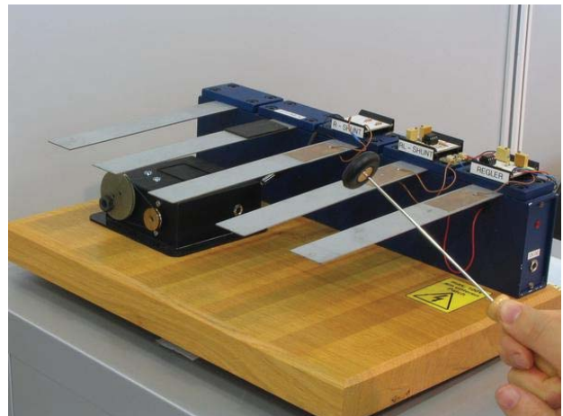
Slika 19. Usporedni test prigušivača [11]
