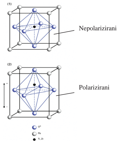
Slika 16. Struktura PZT keramike [9]
