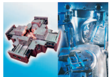
SLIKA 6. Kalupi za tlačni lijev mjenjačke kutije (lijevo) i injekcijsko prešanje spojlera (desno)
