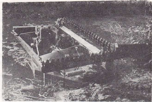
Slika 4. Kosačica za ribnjake »Vihor«, prva domaća kosačica vodene flore proizvođača »Gramip« iz Dubrave
