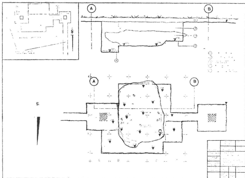
4. Goričan 83 — tlocrt poluzemuničnog objekta položaj »Viko«
