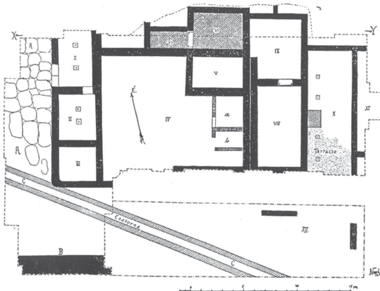
Prilog 2: Tlocrt rimskog vatrogasnog doma (Váry Lászlóne, „Der Feuerwehr in Ungarn bis 1918 ein historischer Abriss“, u katalogu: Burgenländische Landessonderausstellung Feuerwehr gestern und heute, Eisenstadt, 1998.)
