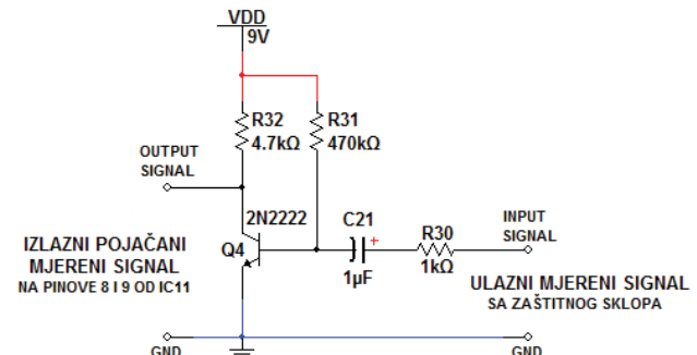
Slika 6. Ulazno pojačalo
