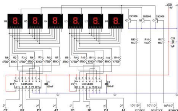
Slika 13. 7-segmentni dekodер и pokazivač
