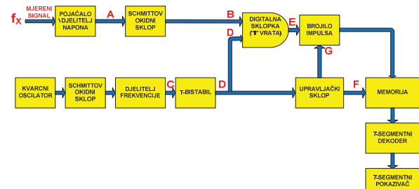
Slika 1. Principijelna blok shema digitalnog frekvencmetra
