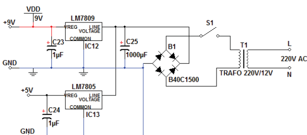
Slika 4. Napajanje
