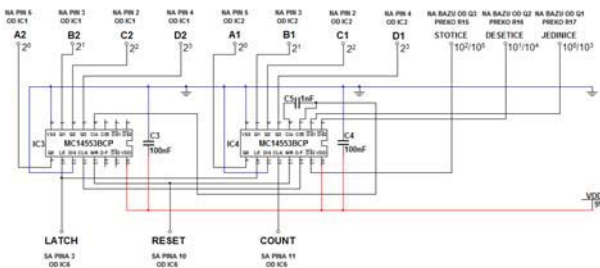
Slika 12. Dekadsko brojilo impulsa
