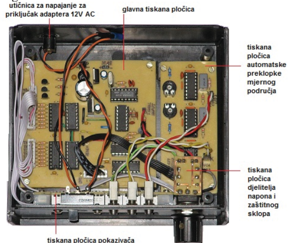
Slika 14. Raspored tiskanih pločica u kućištu digitalnog frekvencmetra
