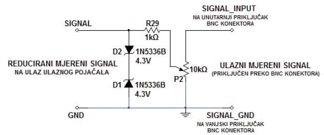
Slika 5. Djelitelj napona i zaštitni sklop
