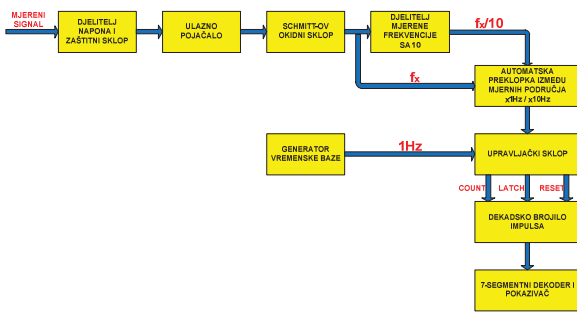
Slika 3. Blok shema izrađenog digitalnog frekvencmetra
