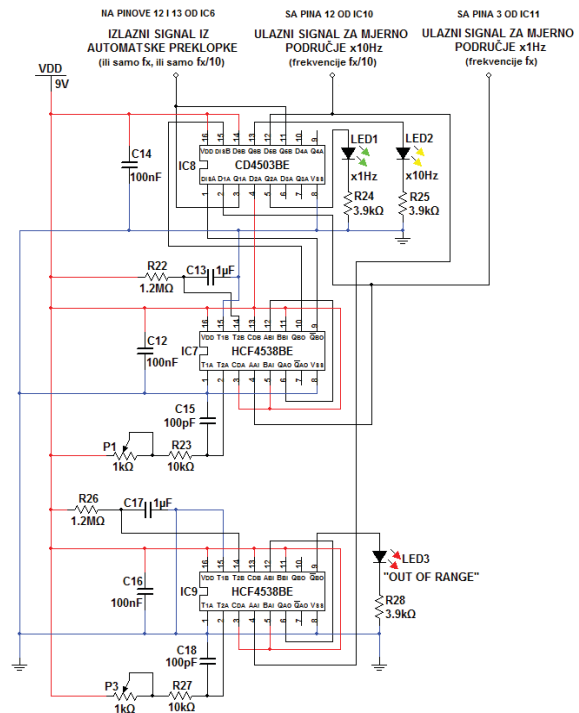
Slika 9. Automatska preklopka između mjernih područja x1Hz i x10Hz
