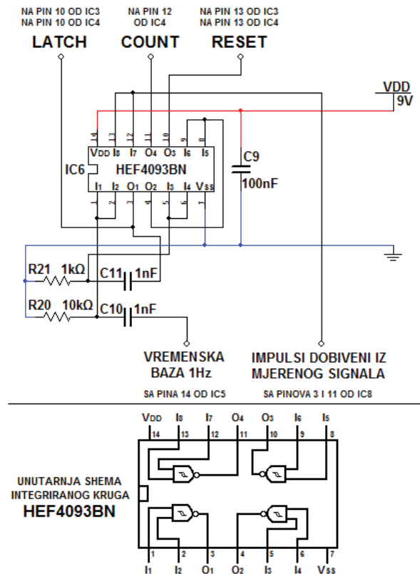
Slika 11. Upravljački sklop
