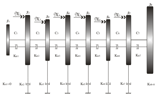
Slika 1. Ekvivalentni dinamički sustav motora SUI
