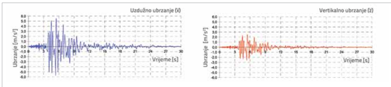
Slika 18. Akceleroogram potresa u Stonu iz 1996. godine
