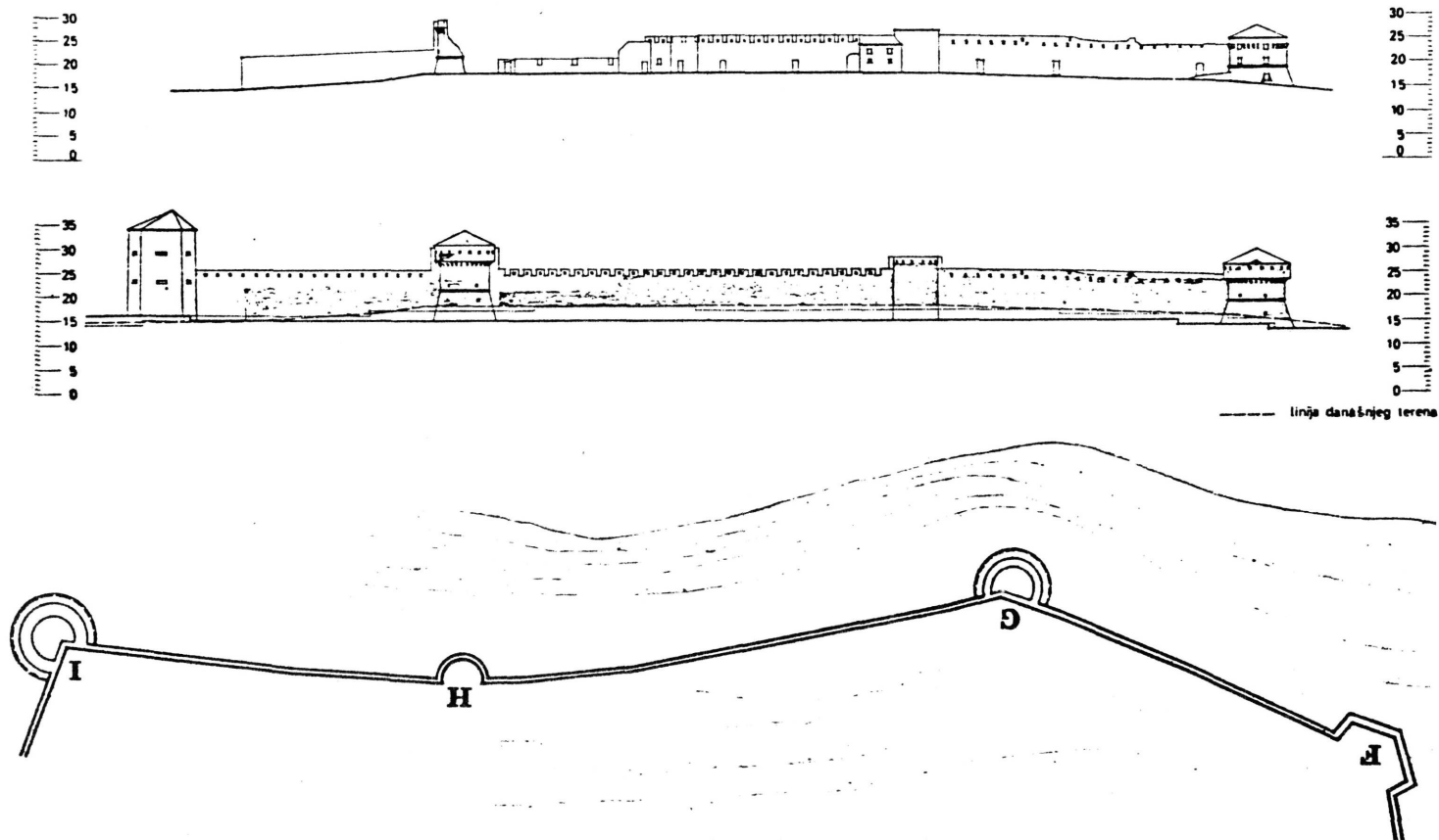
Sl. 17. — Snimak tlocrta postojećeg stanja i grafičke rekonstrukcije sjevernih gradskih zidina i kula Senja u 1 Staroj cesti. Izradila Dr arh. Melita Viličić. 1966. Mjerilo 1 : 500
