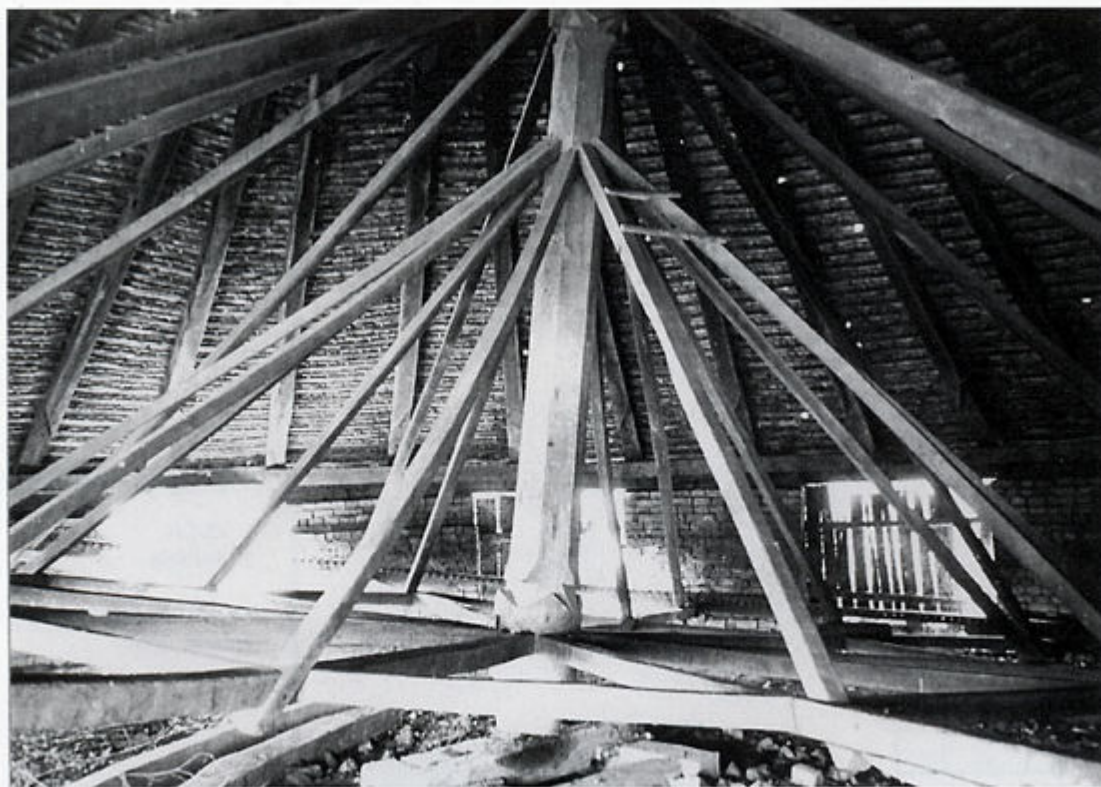
Konstrukcija šatorastog krovista (foto: N. Vranić, 1961.)
