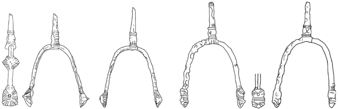
Sl. 12 Ostruge iz Bagruše, identičan par iz Varivoda (Prema: Žeravica 1985-1986; Petrincec 2009 – crteži: N. Šimundić-Bendić)
