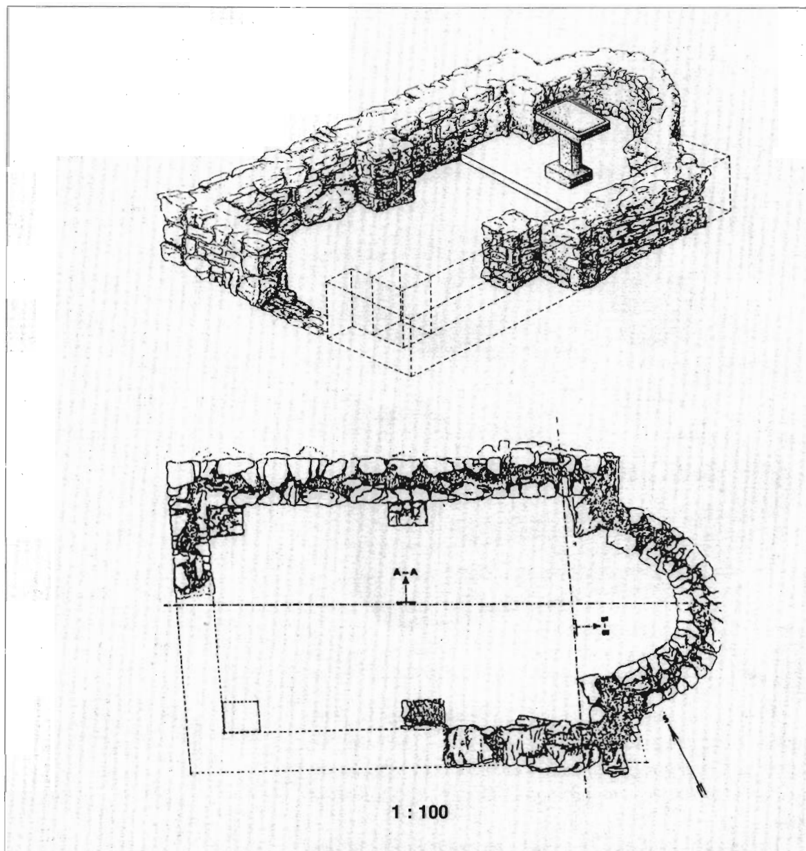
Perspektivni izgled i tloris od crkve Sv. Vida
