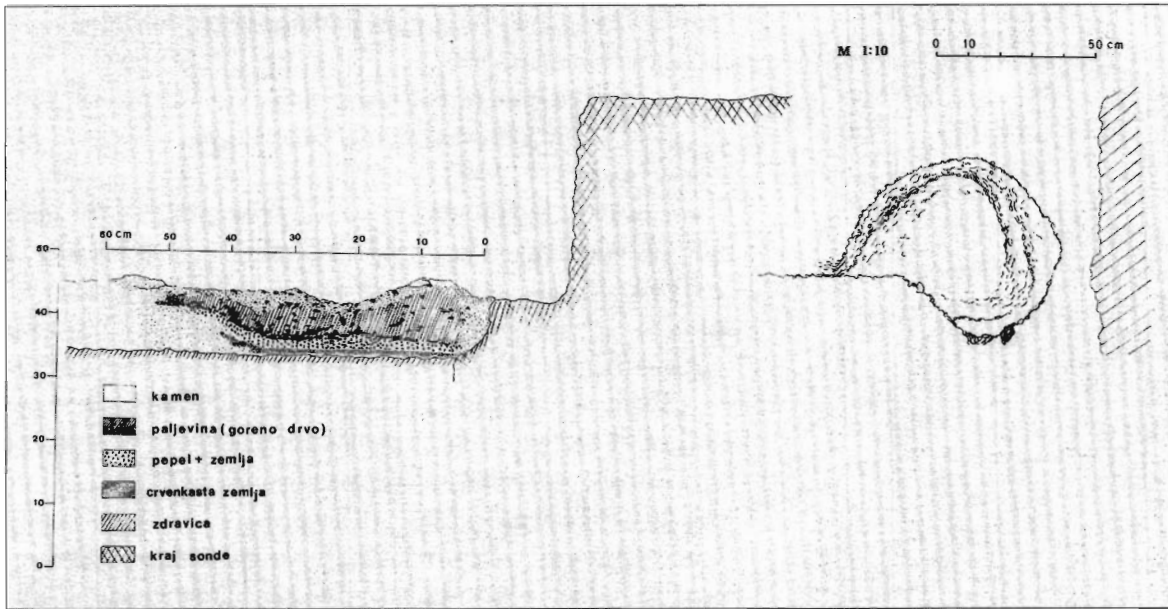
Presjek i tlocrt jame s paljevinom na položaju Gluvinih kuća II
