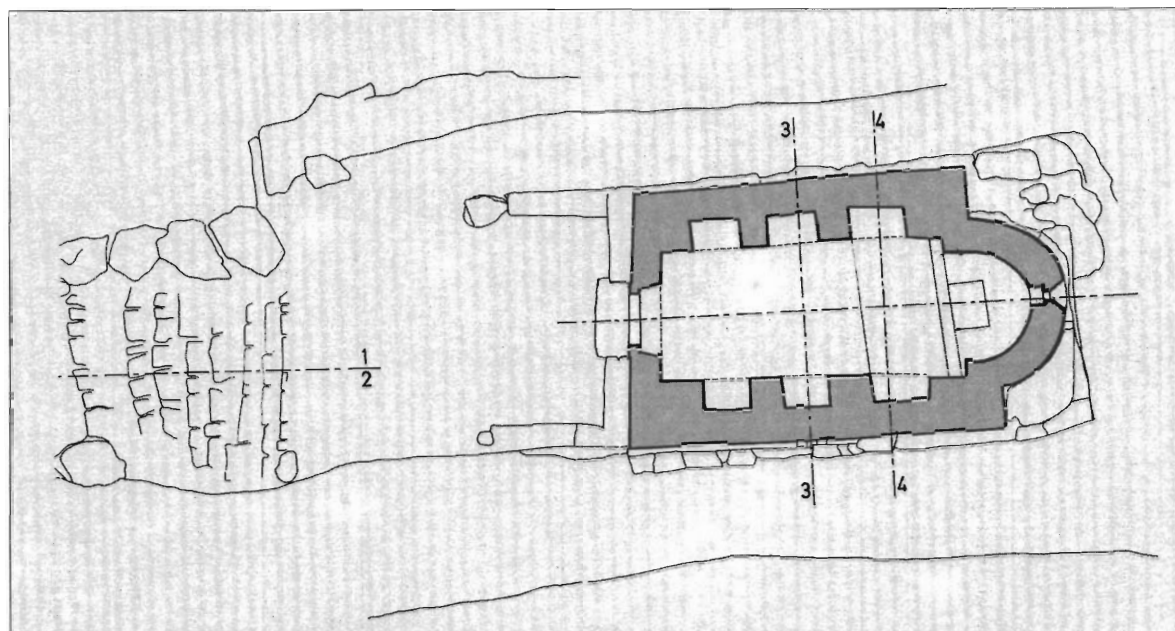
Tlocrt crkve Sv. Mihovila i užeg okoliša crkve
