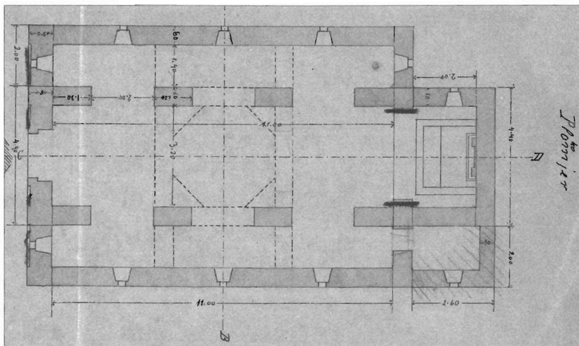
Prijedlog rekonstrukcije tlocrta ranosrednjovjekovne crkve Sv. Marte, prema ideji inž. A. Bezića, 1902. godine.
