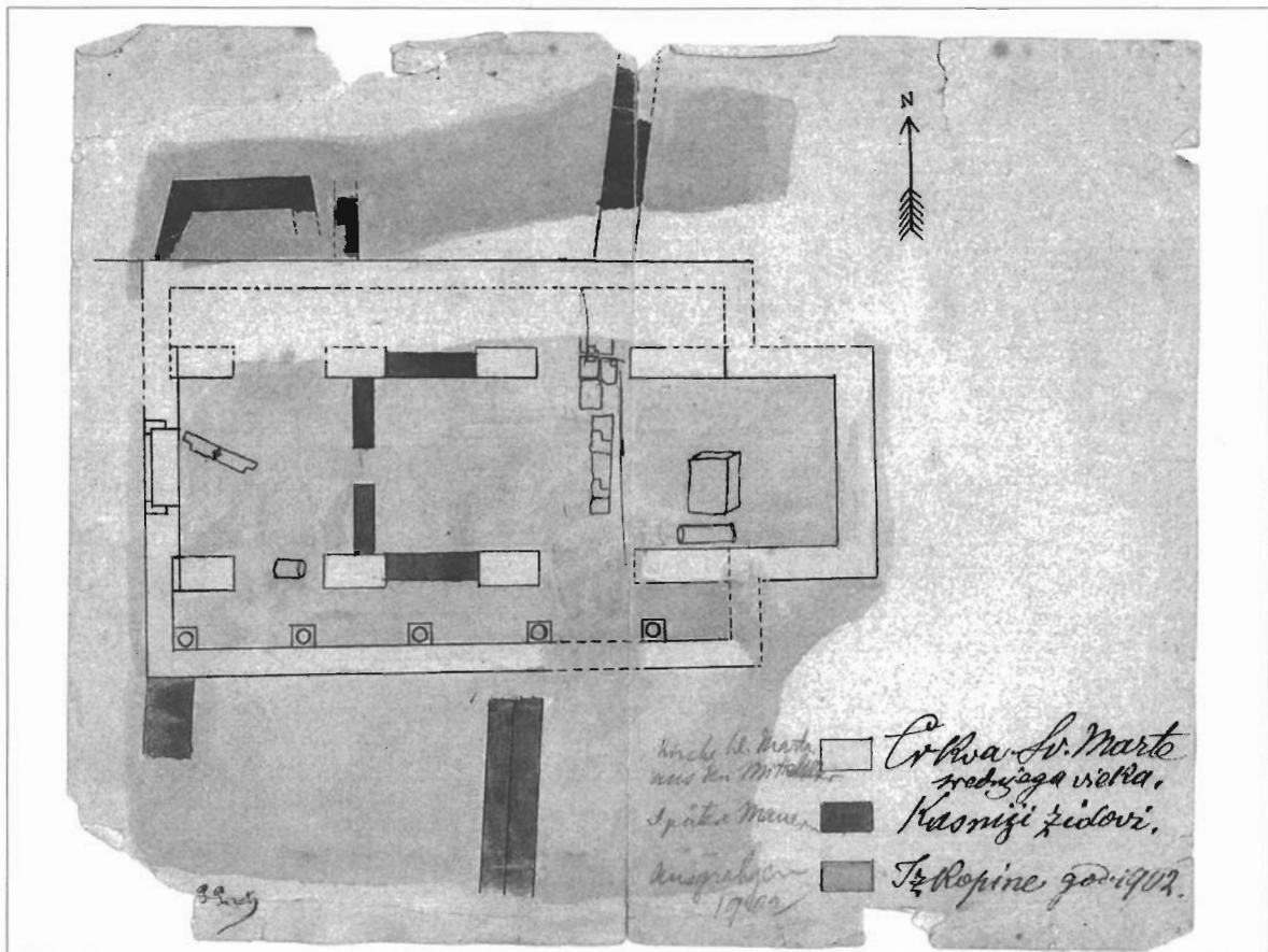
Tloris otkopanih zidova kod crkve Sv. Marte 1902. godine.
