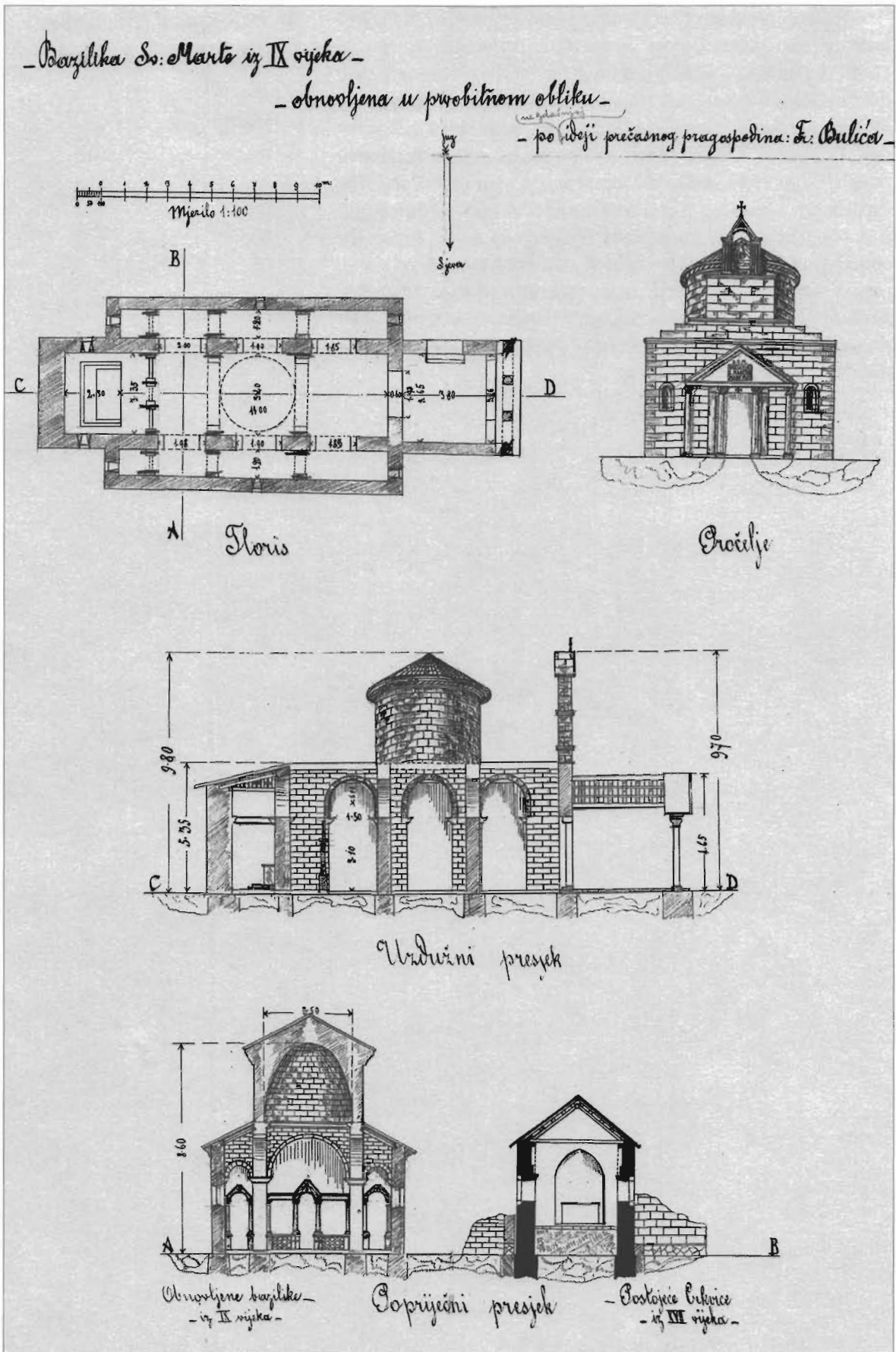
Prijedlog rekonstrukcije ranosrednjovjekovne crkve Sv. Marte, prema ideji don. Frane Bulića.
