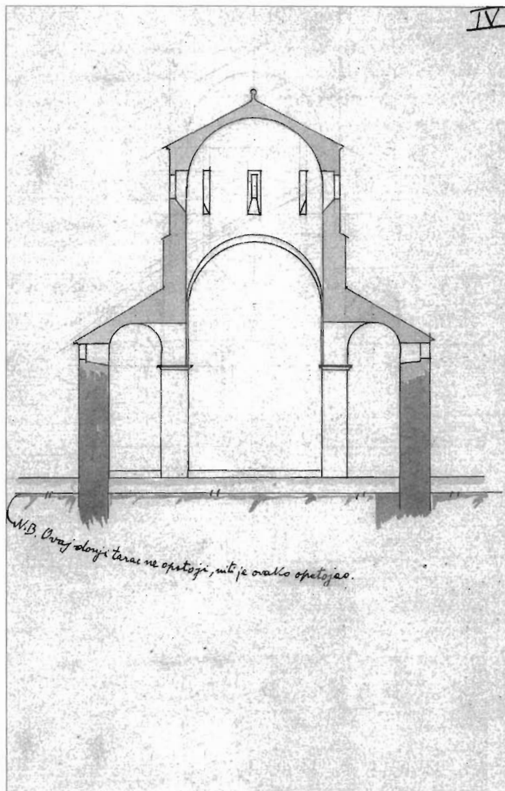
Pretpostavljeni izgled poprečnog pres- jeka ranosrednjovjekovne crkve Sv. Marte.
