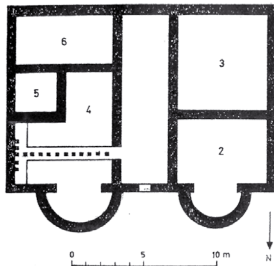
7. Tlocrt i rekonstrukcija dvoapsidalne građevine iz Keszthely-Fenekpuszta (izvor: THOMAS, E. B., 1980., 300-301)
