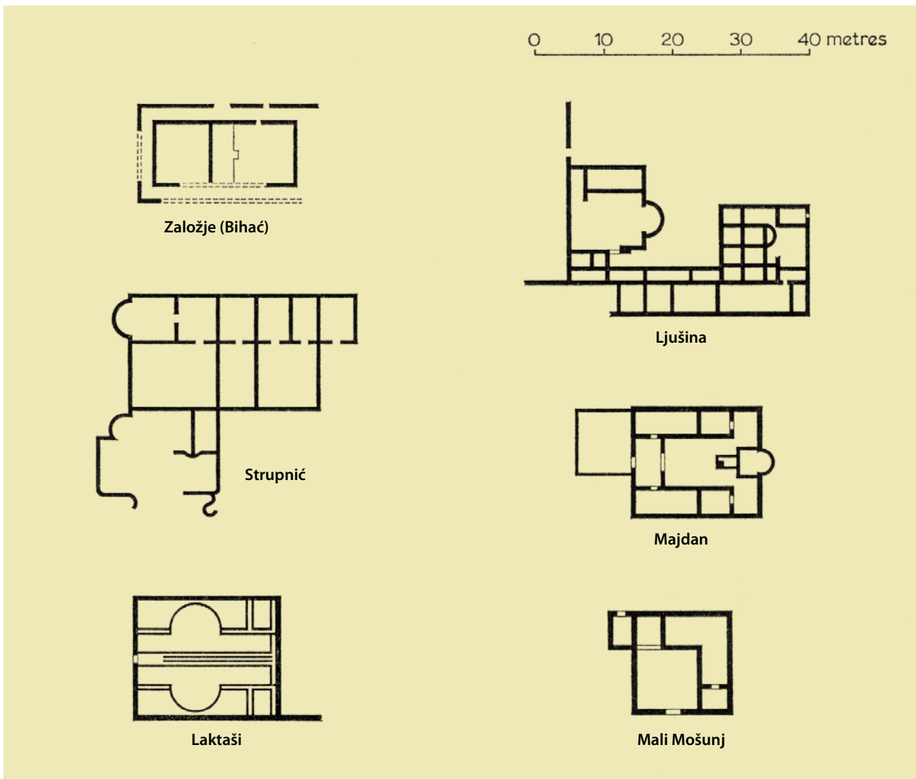
3. Wilkesove usporedbe vila iz dalmatinske unutrašnjosti (izvor: WILKES, J. J., 1969., 404)
