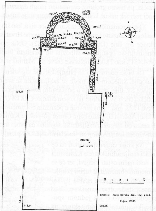
Sl. 3: Kamešnica, gotička crkva Sv. Andrije, apsida i lađa romaničke crkve (tlocrt), te grobovi
