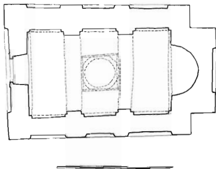
Sl. 7. Tlocrt, pretpostavljeno izvorno stanje
