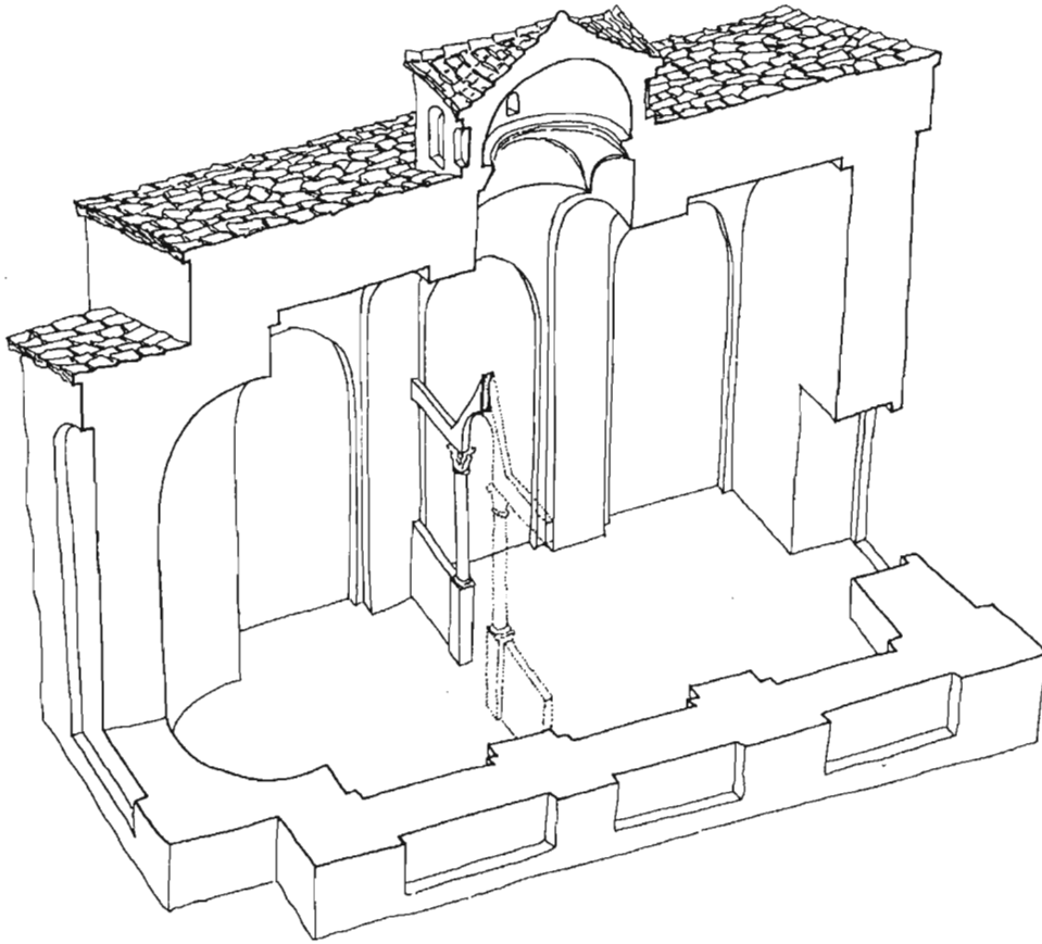
Sl. 10. Perspektivni prikaz unutrašnjosti crkve
