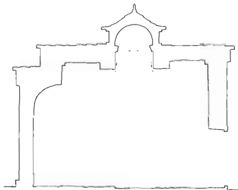
Sl. 8. Presjek, pogled sjever, pretpostavljeno izvorno stanje
