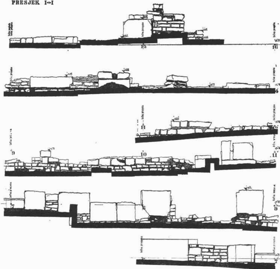
Sl. 4. Južna crkva, presjek I—I. — Südlische Kirche, Querschnitt I.—I.
