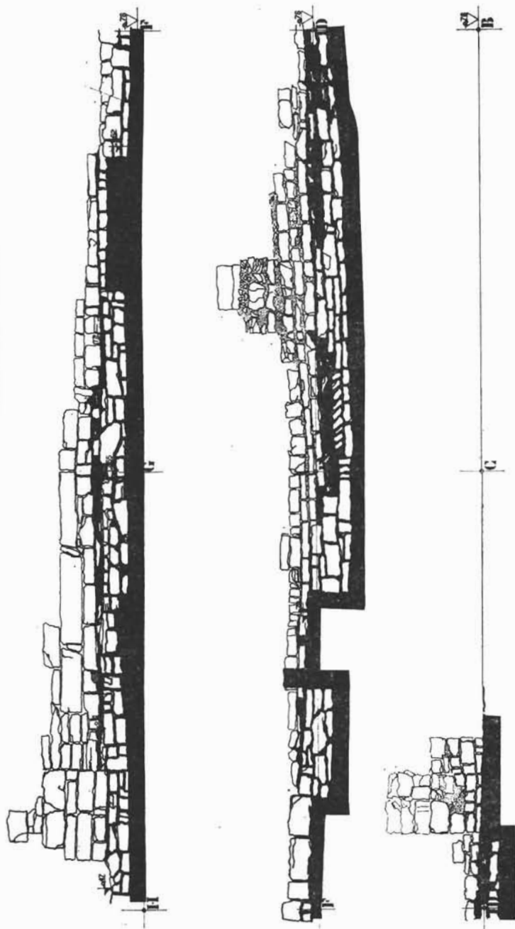
Sl. 1. Južna crkva, presjek VII-VII. — Südliche Kirche, Querschnitt VII.—VII.
