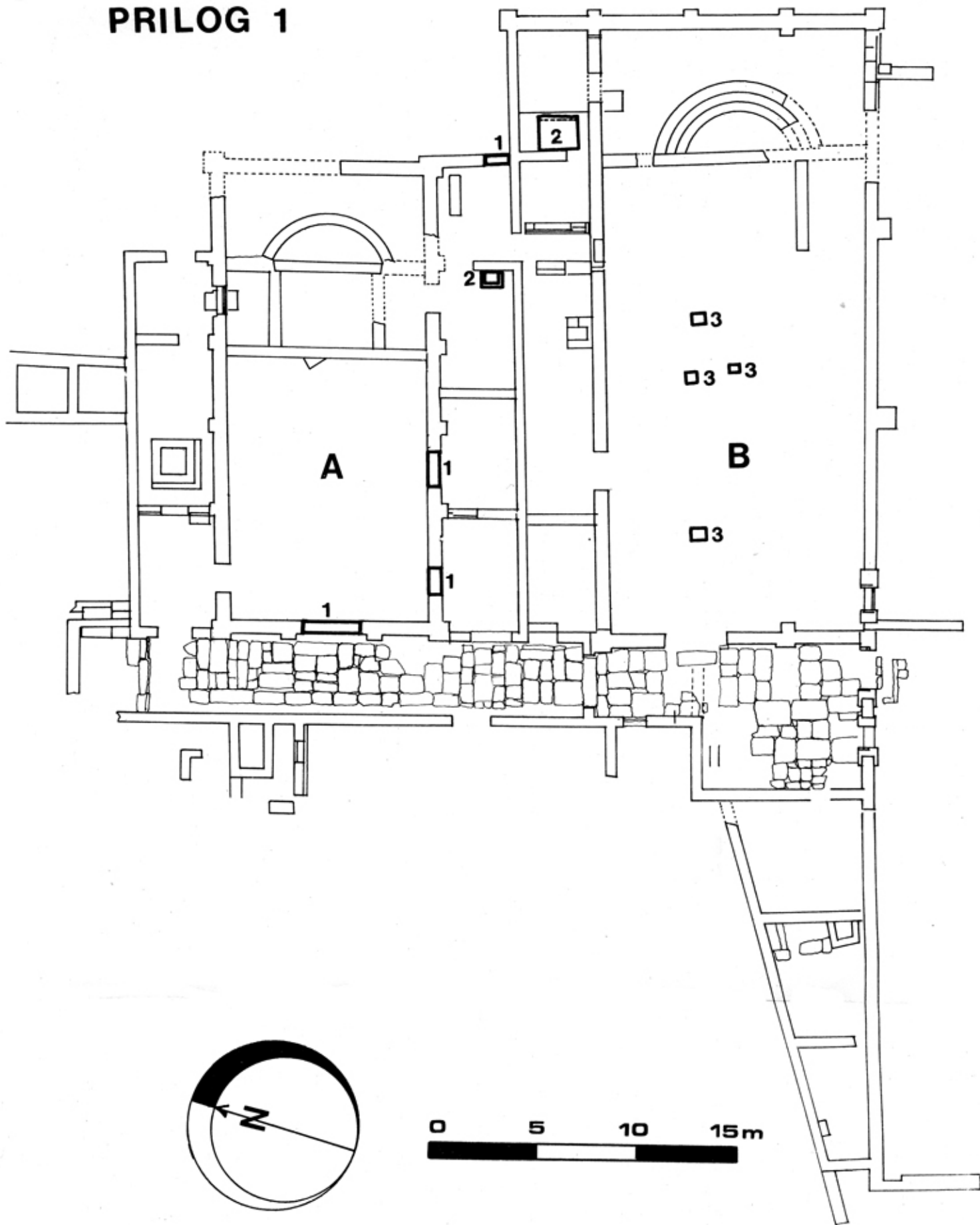
Prilog 1. Bazilika gemina, tlocrt (prema A. Puschiju). Legenda: A = sjeverna crkva, B = južna crkva, 1 = zazidani ulazi, 2 = ognjišta, 3 = nepravilno razmještene grupe kamenja. — Basilica gemina, Grundriß (nach A. Pusch). Legende: A = nördliche Kirche, B = südliche Kirche, 1 = zugemauerte Eingänge, 2 = Herdstellen, 3 = unregelmäßige Steinhaufen
